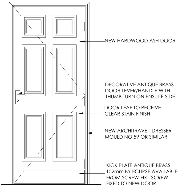
DOOR TYPE B - EN-SUITE DOORS
