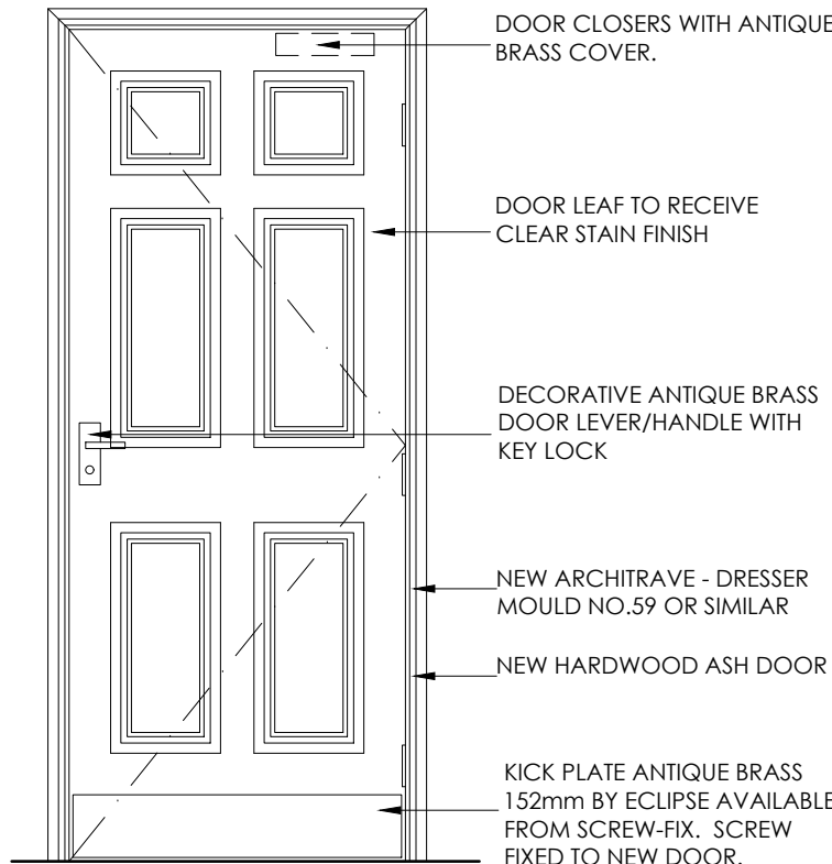
DOOR TYPE D - GENERAL DOORS
