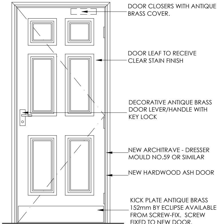
DOOR TYPE A - BEDROOM DOORS
