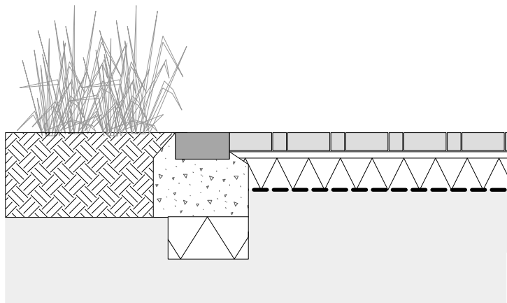
1 E1 Concrete Planting Edge Scale: 1:25
