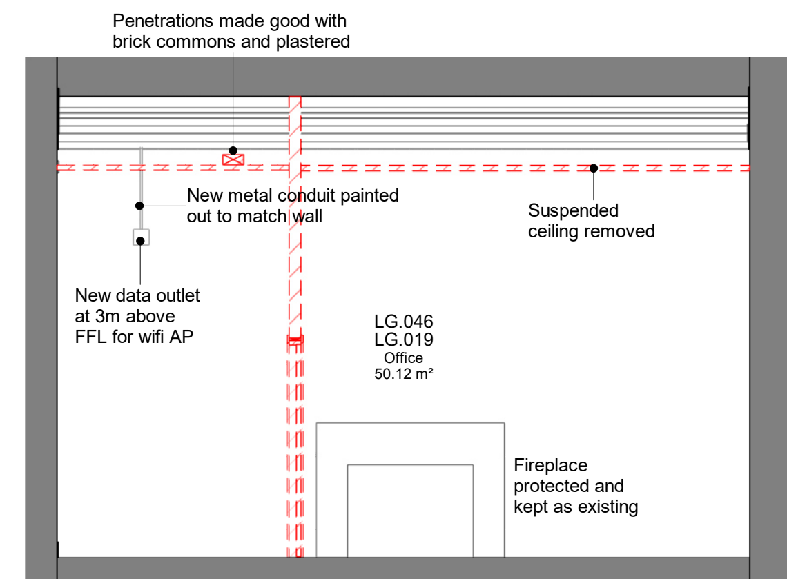
LG.019 Elevation D
