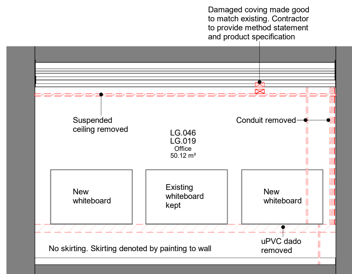
LG.019 Elevation B
