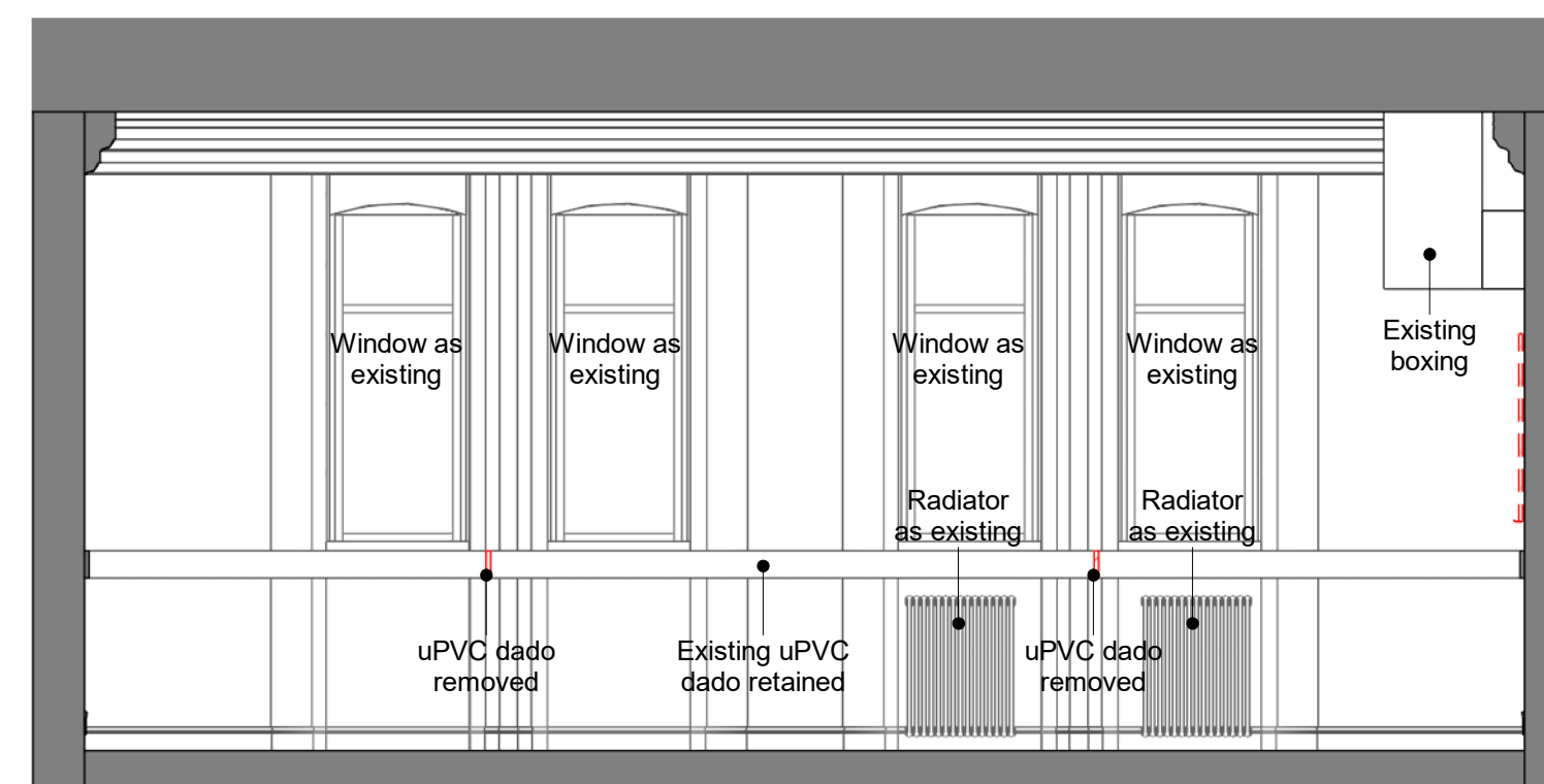
LG.005 Elevation E
