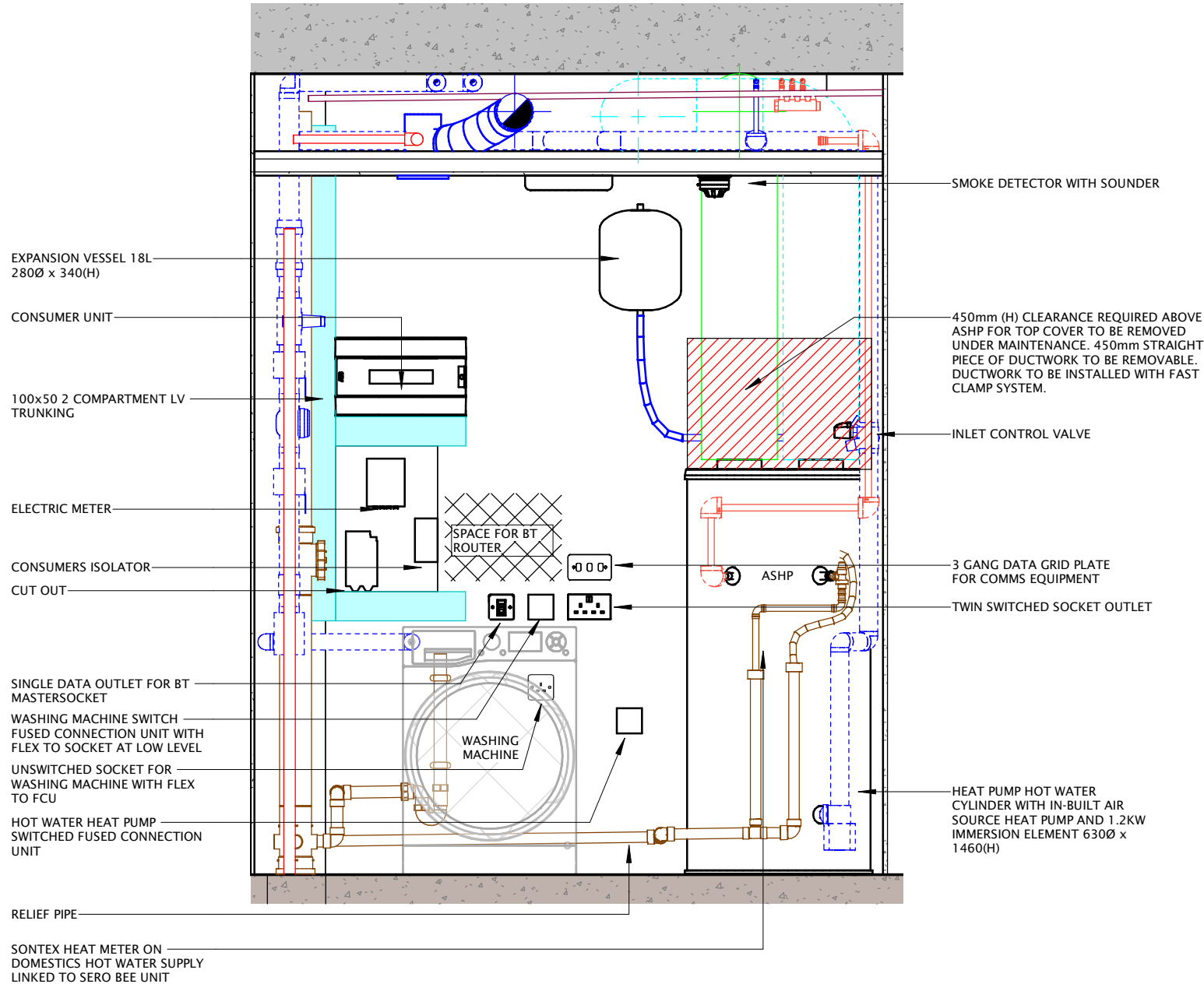
Type 01 - Elevation A 1 : 20
