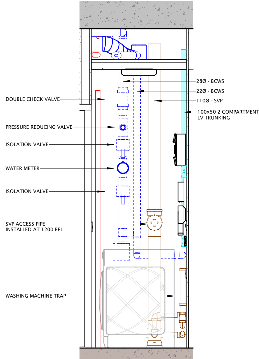
Type 01 - Elevation D 1 : 20
