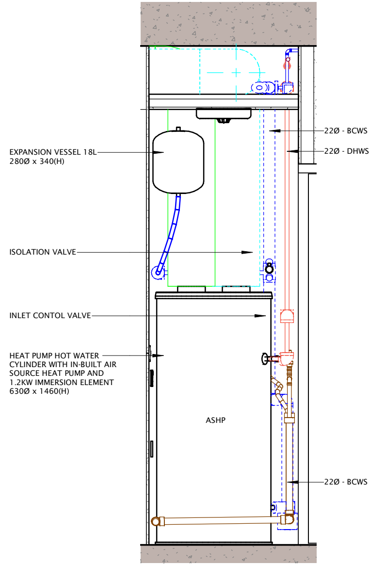
Type 01 - Elevation B 1 : 20
