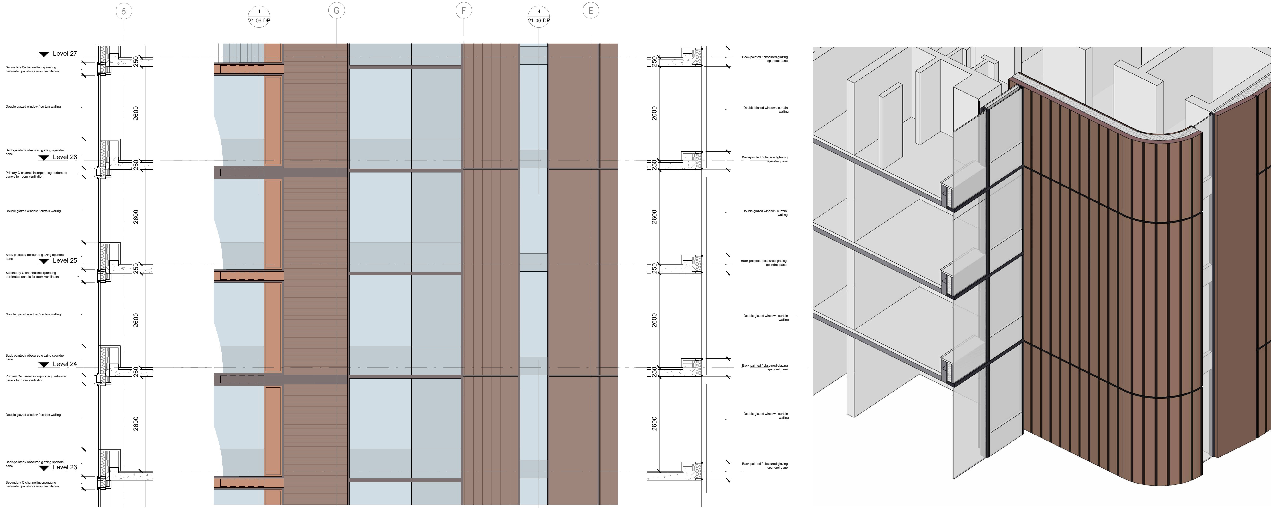
1 Section - Cladding Type 3A 1 : 50
