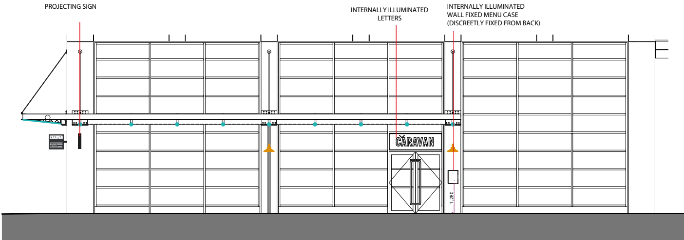
ELEVATION A-A - 1:150
