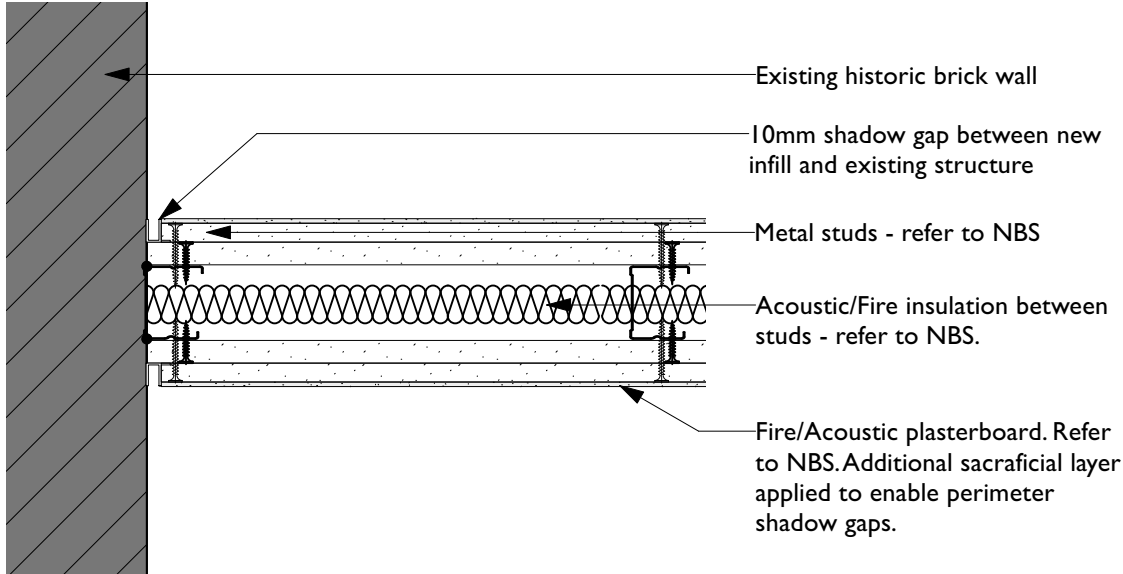
1 Partition Type A Scale: 1:5
