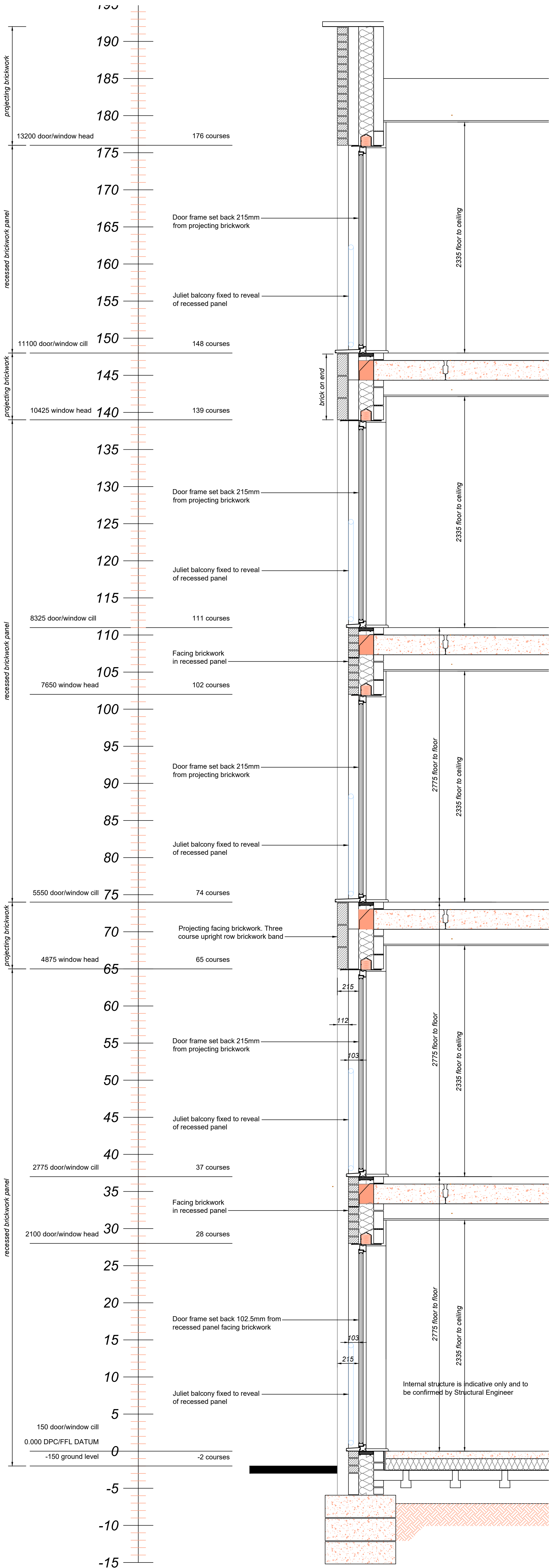
Section A-A
