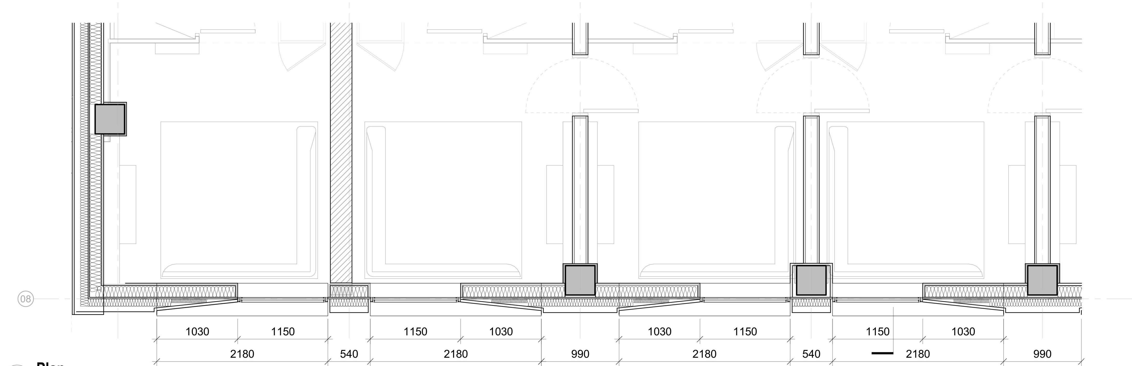
3 Plan 1:25
