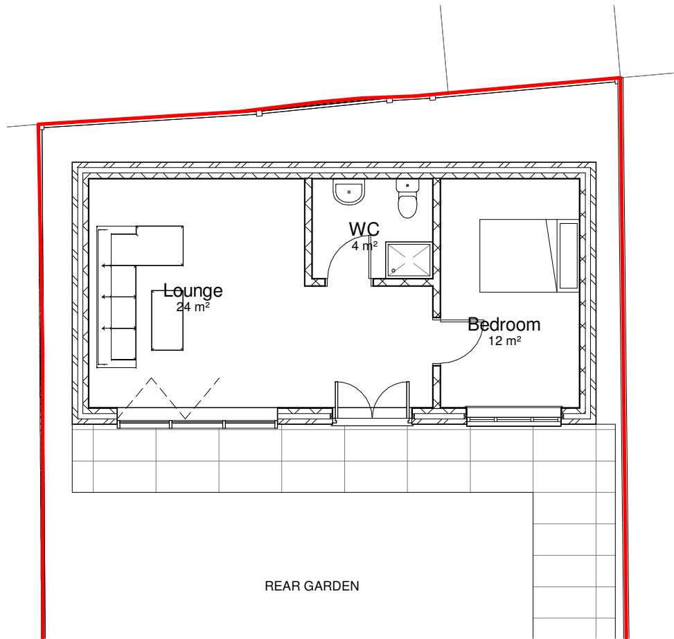
1 Floor Plan 1 : 100
