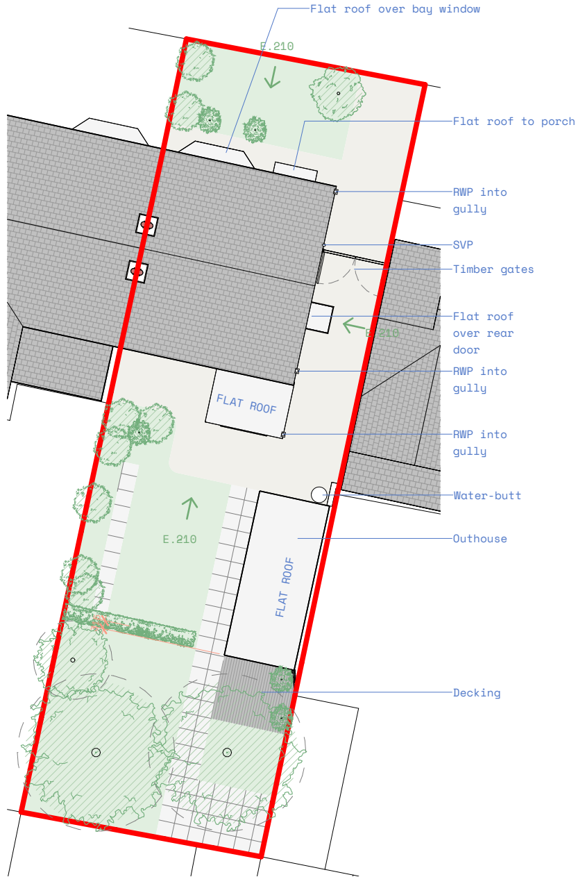
Existing Site Layout Plan 1 : 200
