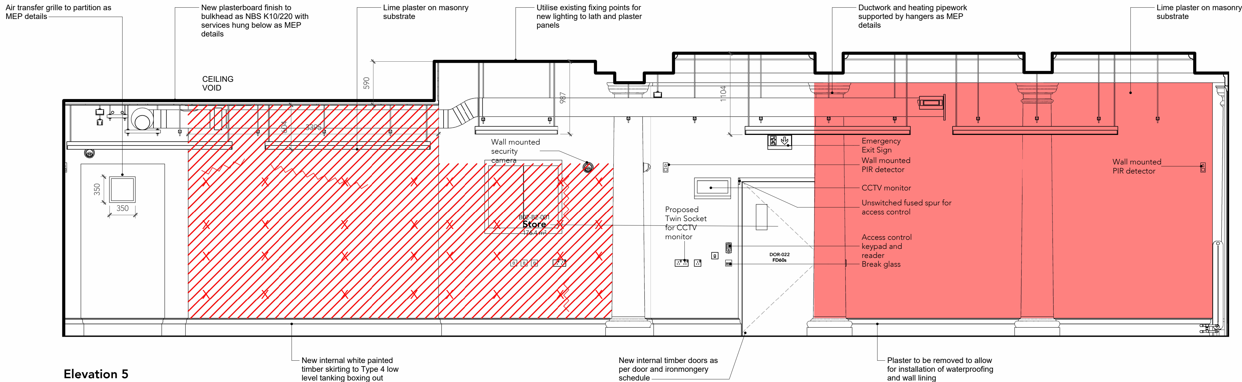
Elevation 5
