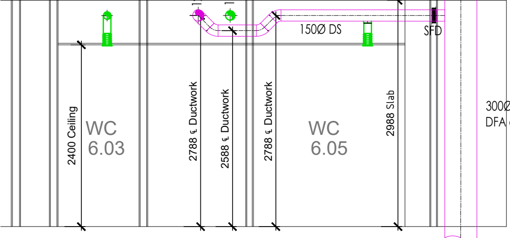
SECTION ON 'B' - 'B' Scale 1:50
