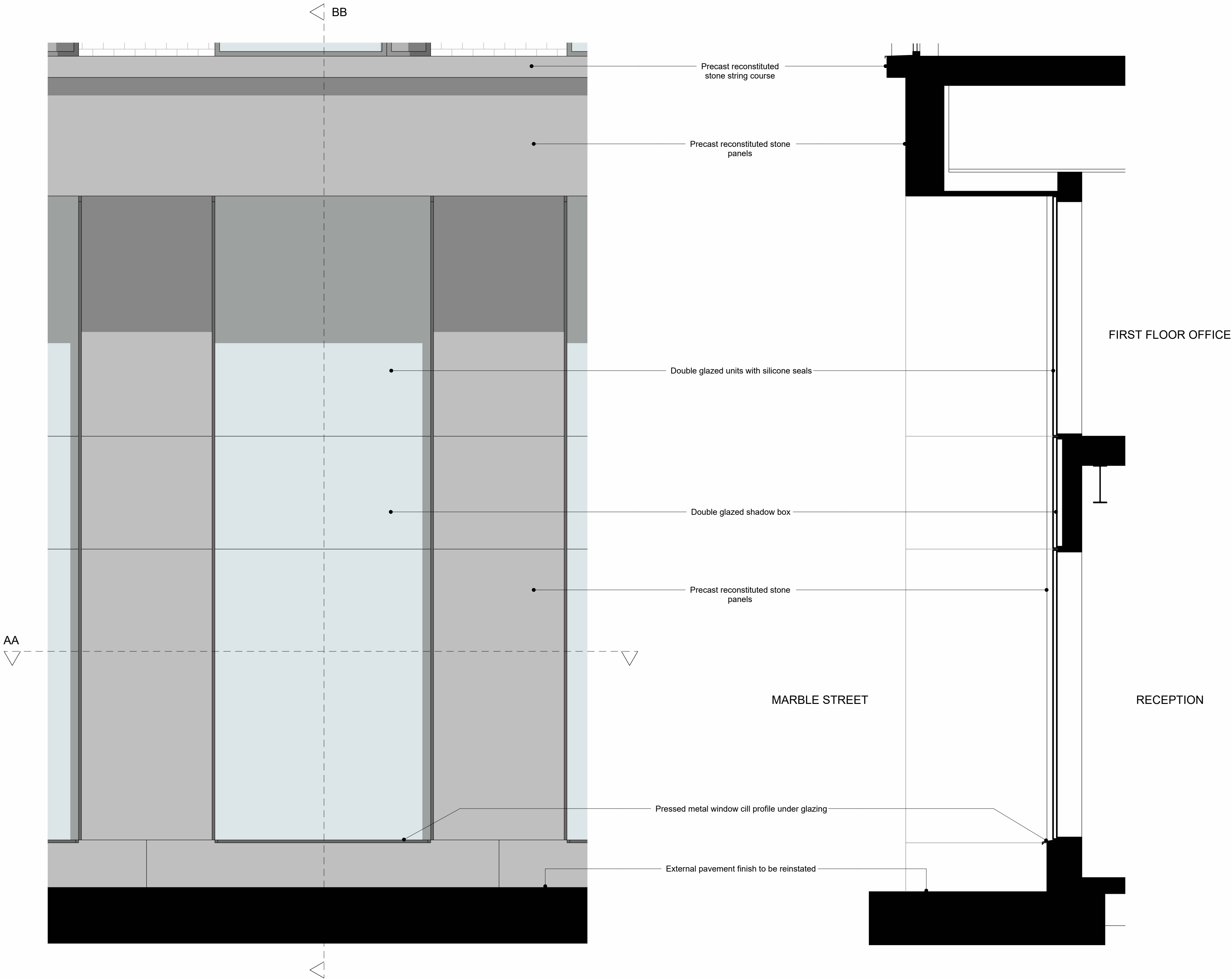
ELEVATION
