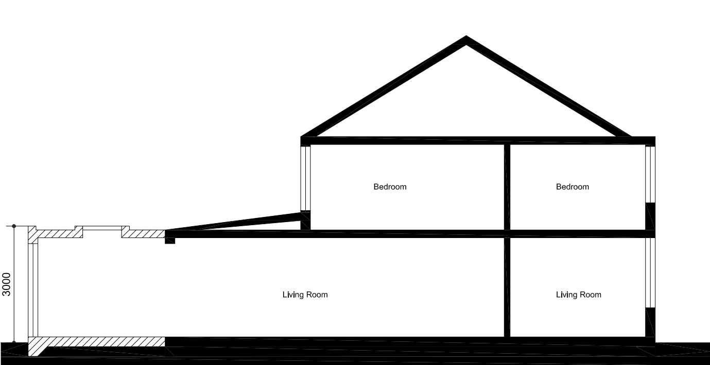
Section 01
