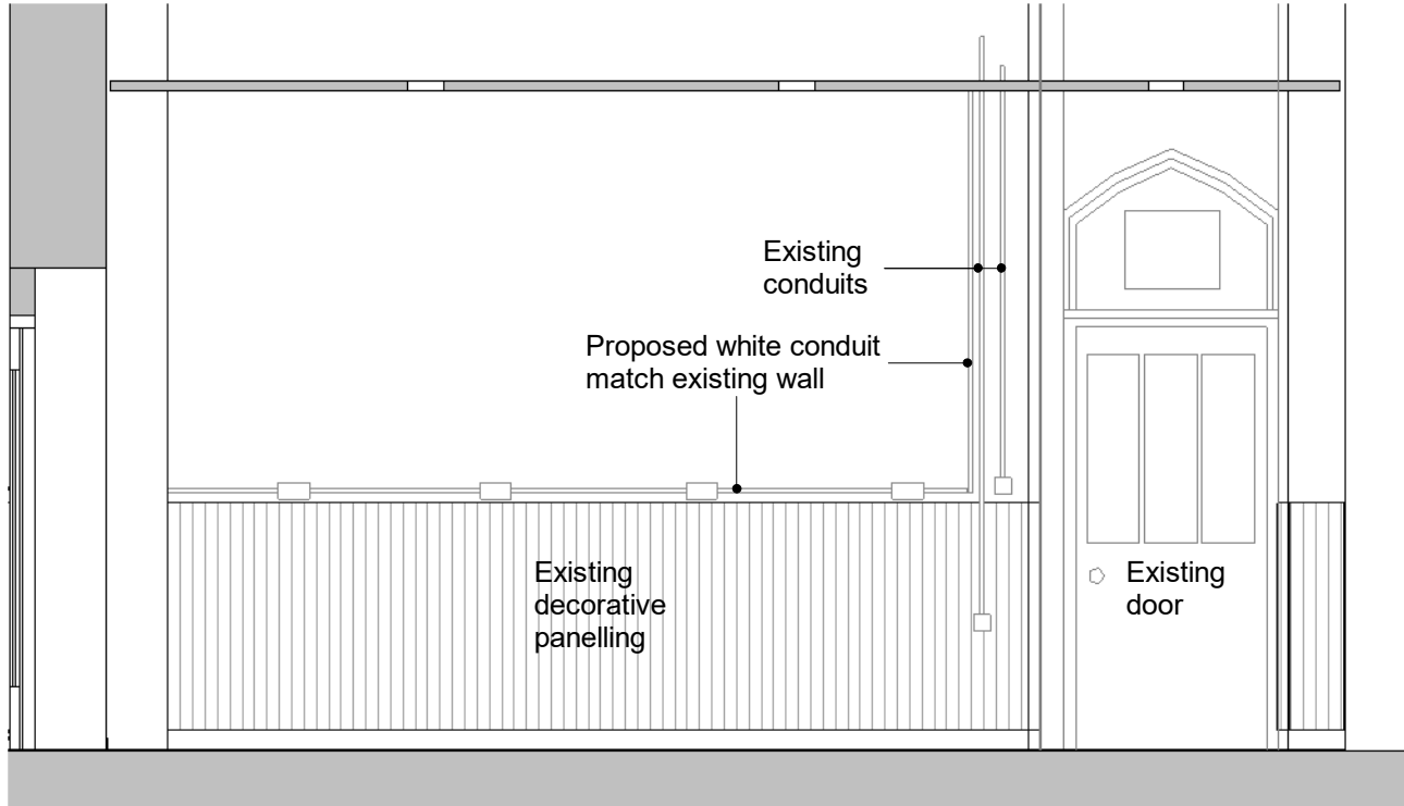
Elevation B
