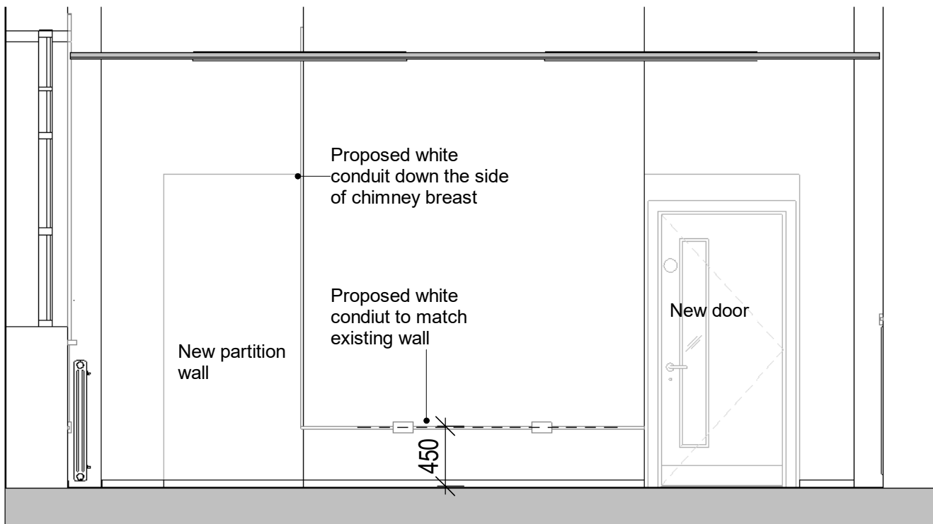
Elevation A
