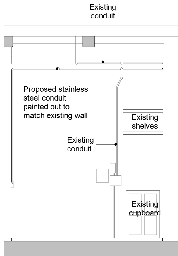
Elevation I
