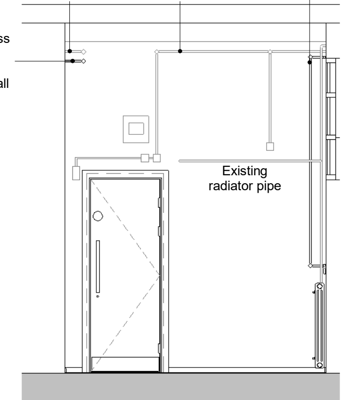
Elevation J
