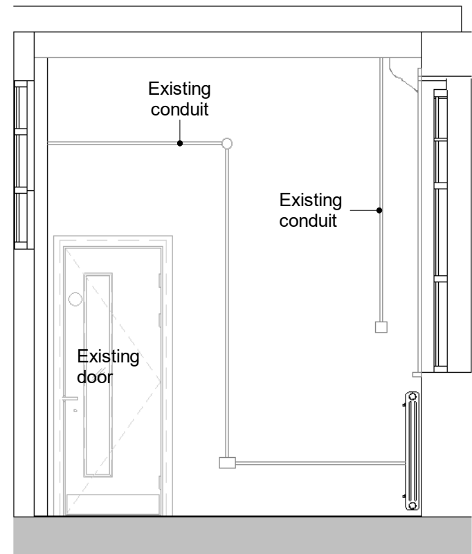
Elevation G
