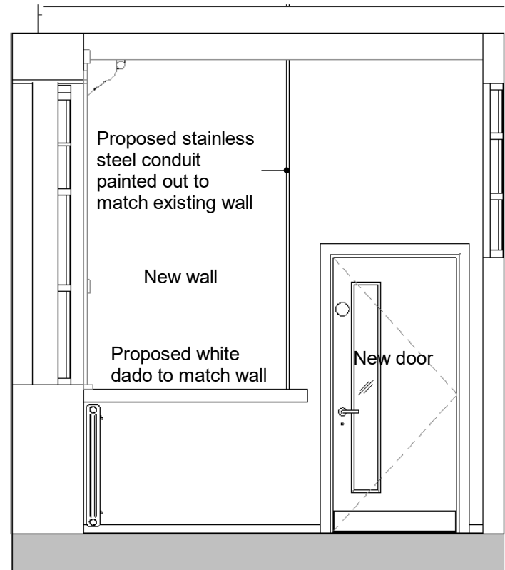
Elevation E
