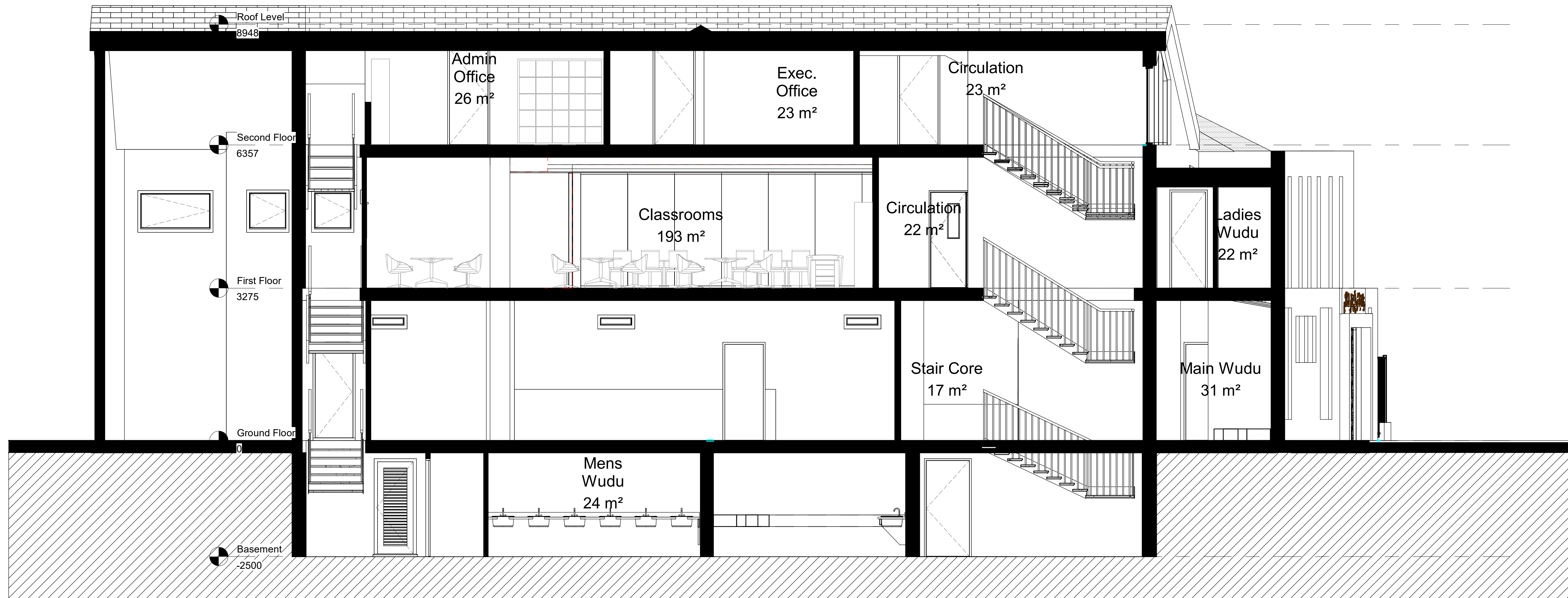
1 Section A-A 1 : 50
