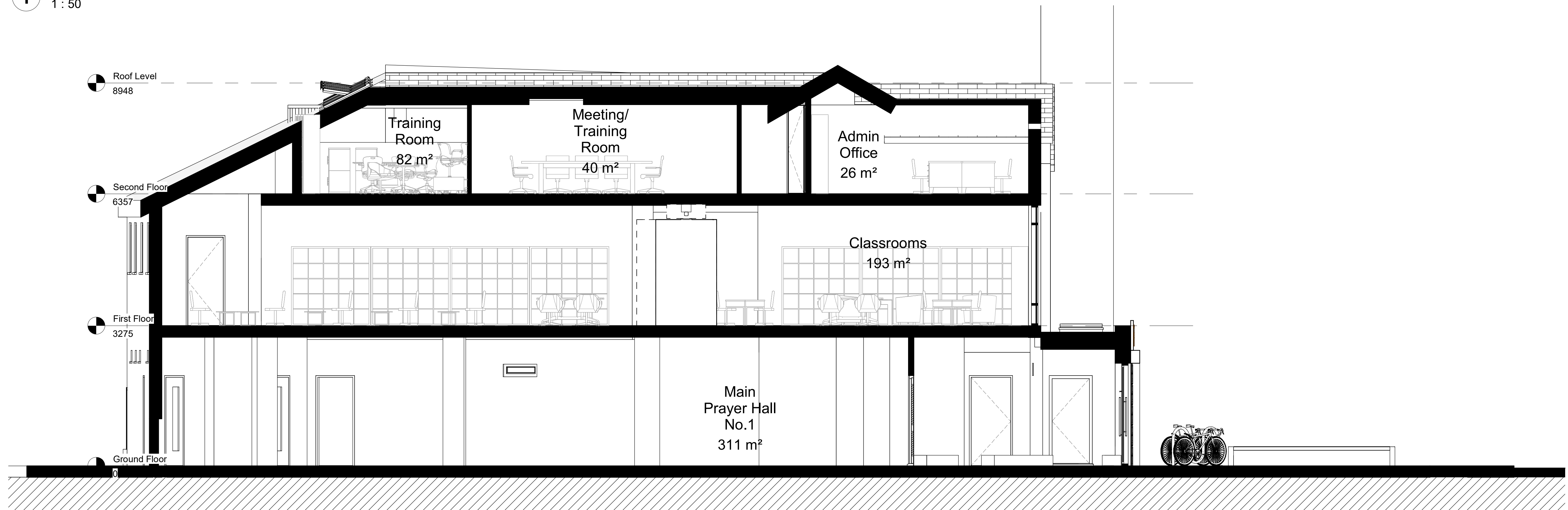
2 Section B-B 1 : 50
