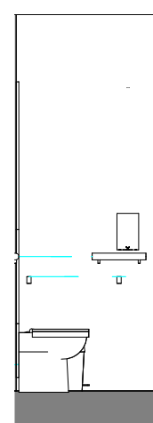
7 ELEVATION 7 1:50
