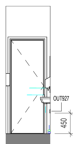
8 ELEVATION 8 1 : 50
