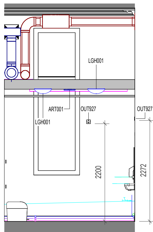
2 ELEVATION 2 1:50
