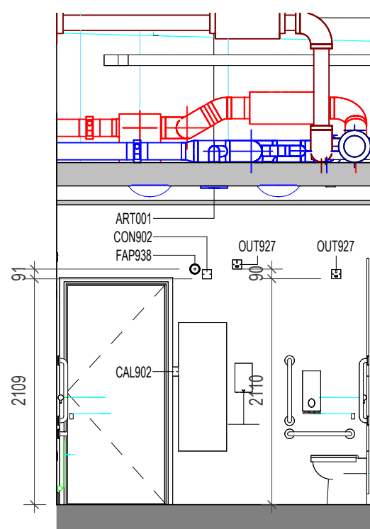
4 ELEVATION 4 1 : 50
