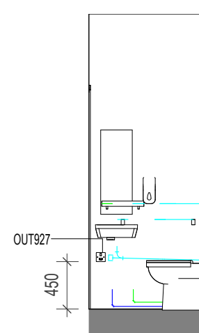
9 ELEVATION 9 1 : 50
