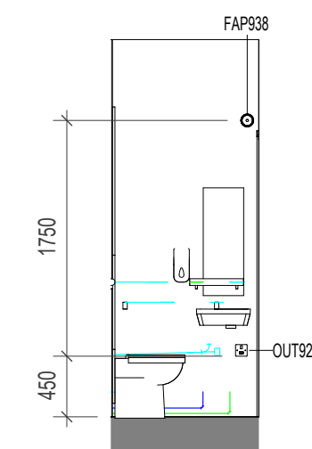
11 ELEVATION 11 1:50
