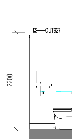
「13」 ELEVATION 13 1:50
