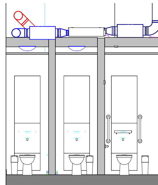
10 ELEVATION 10 1:50
