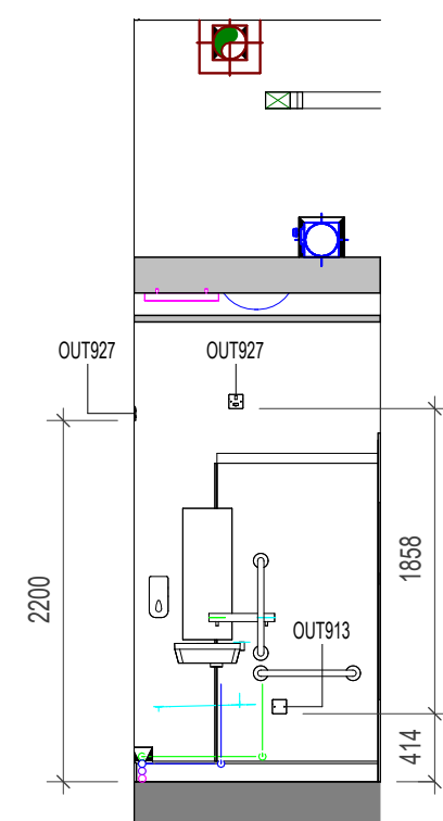
3 ELEVATION 3 1 : 50
