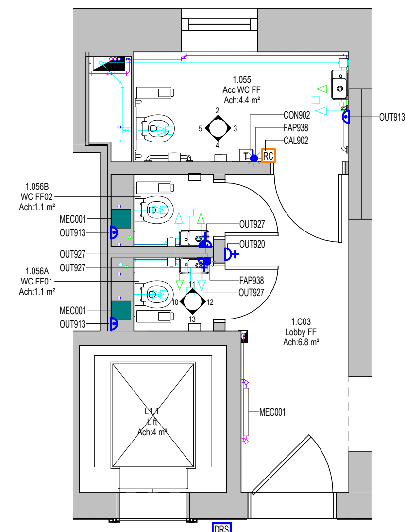
1 1.056 WCs Floor Plan 1 : 50
