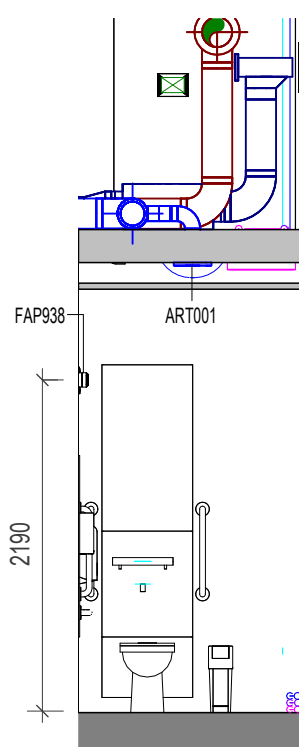
5 ELEVATION 5 1:50
