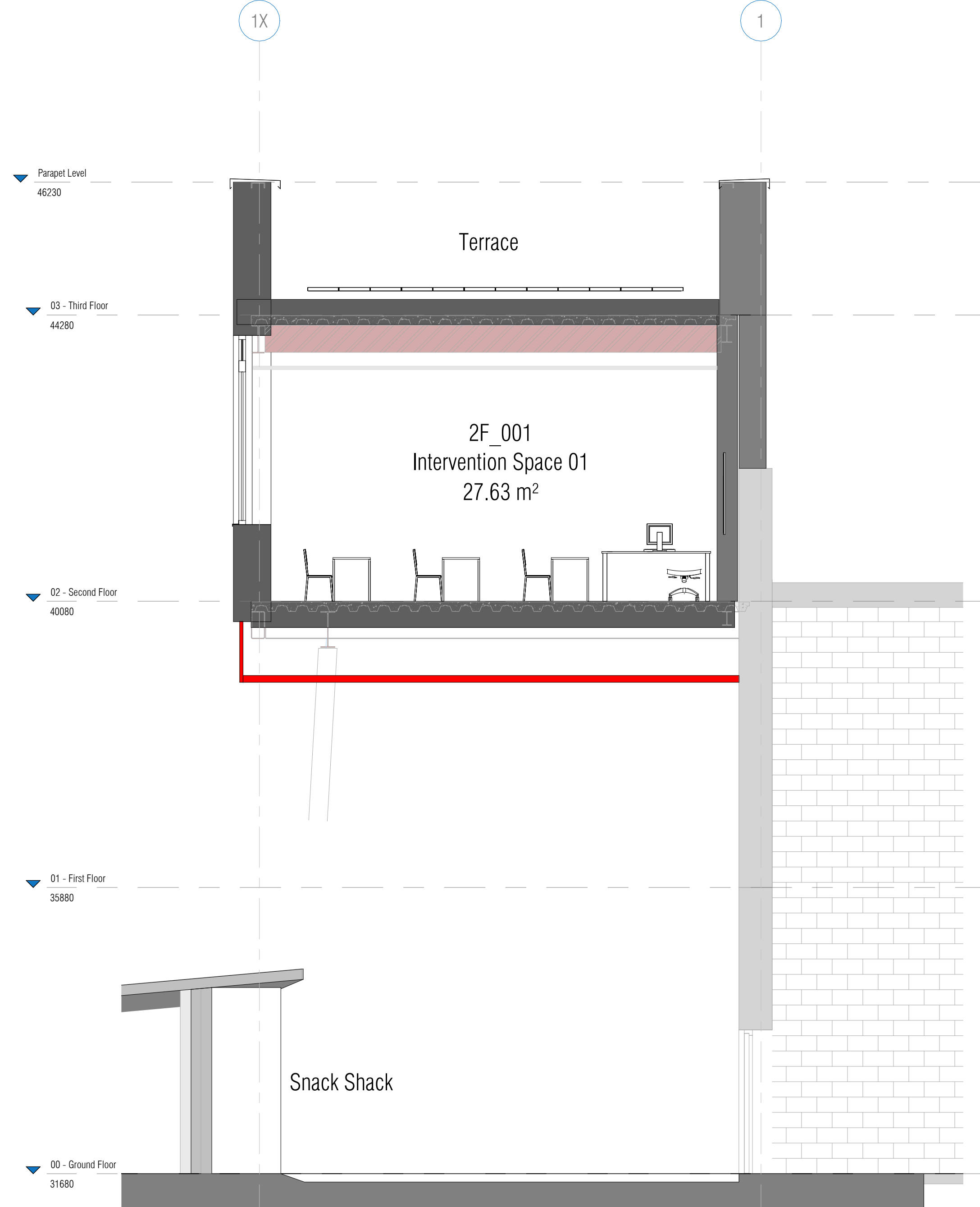
D Section D-D Planning 1 : 50
