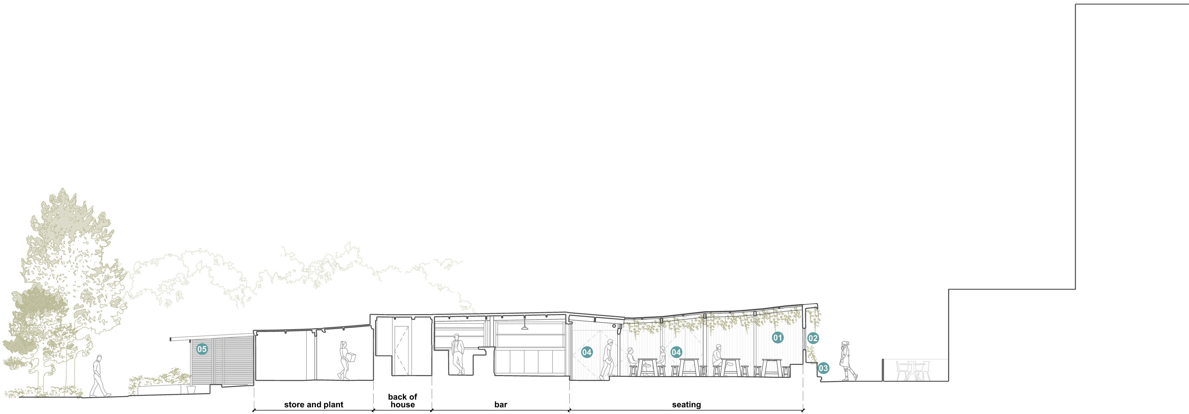
SECTION A-A 1:100 @ A1
