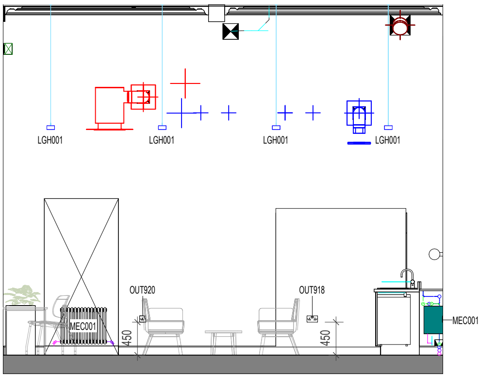
4 ELEVATION 4 1 : 50
