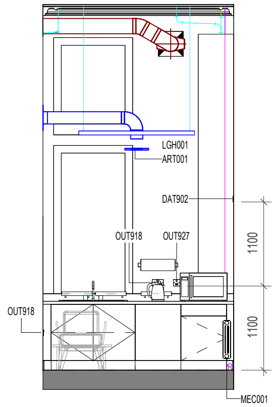
5 ELEVATION 5 1 : 50
