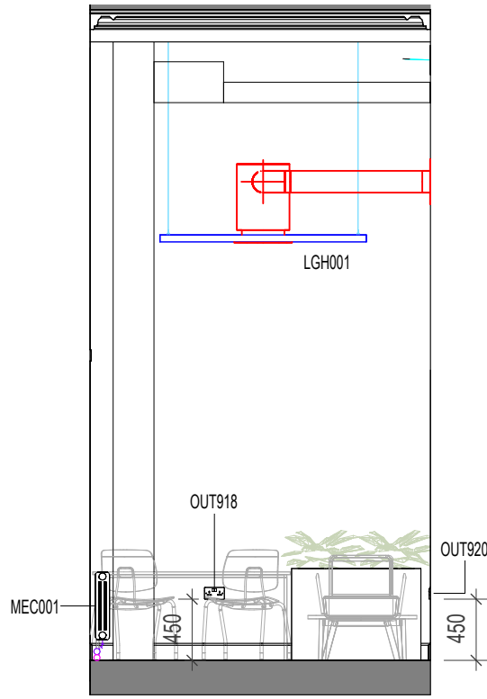
3 ELEVATION 3 1 : 50
