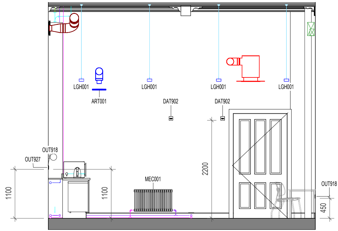
2 ELEVATION 2 1 : 50
