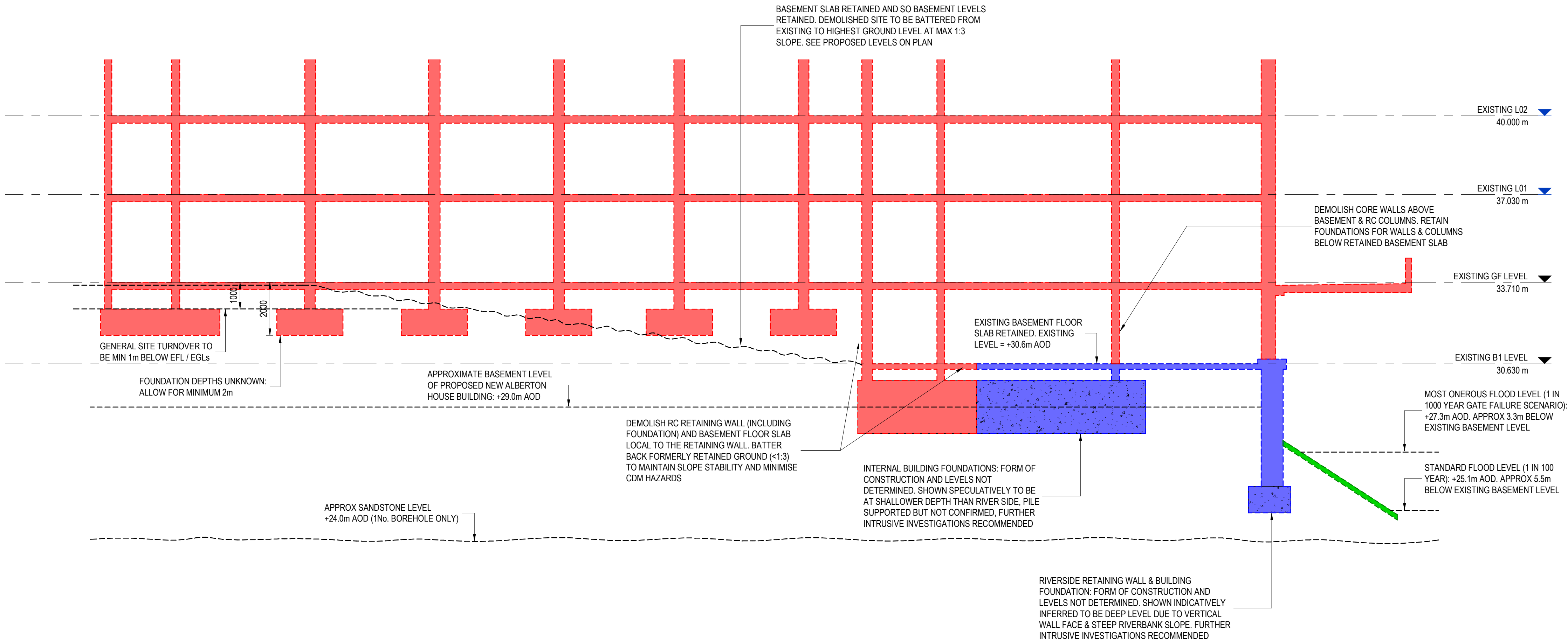
DEMO SECTION 1-1 SCALE: 1 : 100
