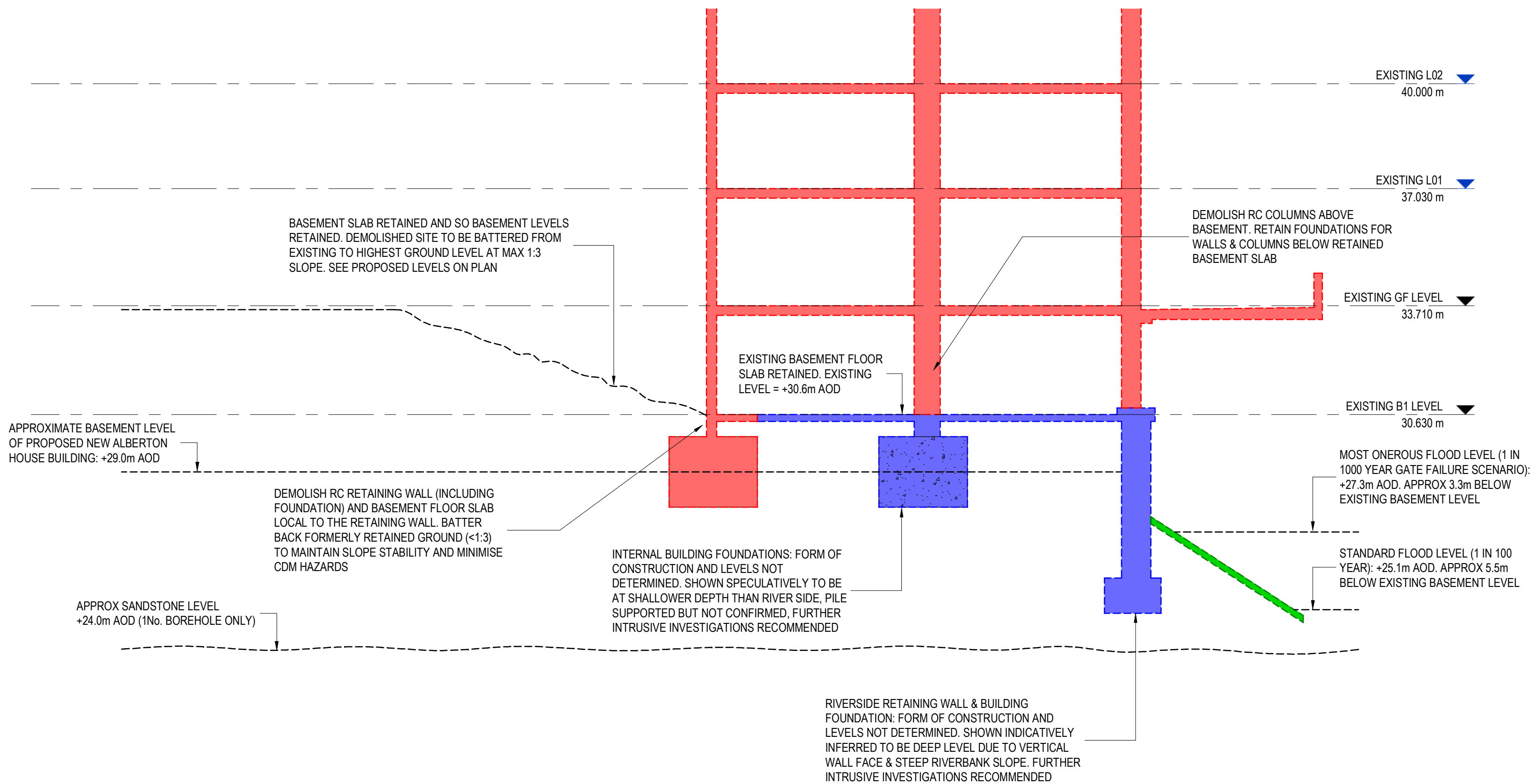
DEMO SECTION 2-2 SCALE: 1 : 100
