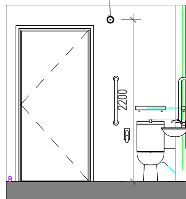
6 ELEVATION 6 1 : 50
