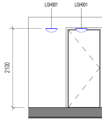
8 ELEVATION 8 1 : 50
