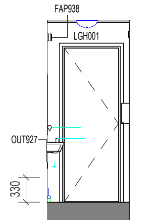
22 ELEVATION 22 1 : 50
