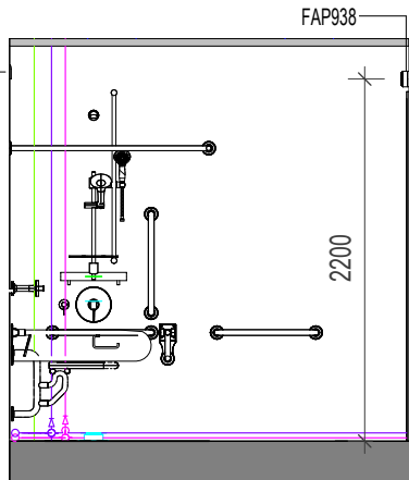
5 ELEVATION 5 1 : 50
