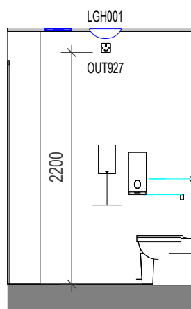
19 ELEVATION 19 1 : 50
