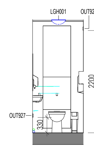
18 ELEVATION 18 1 : 50
