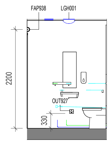
17 ELEVATION 17 1 : 50
