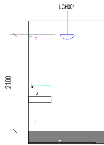
7 ELEVATION 7 1 : 50
