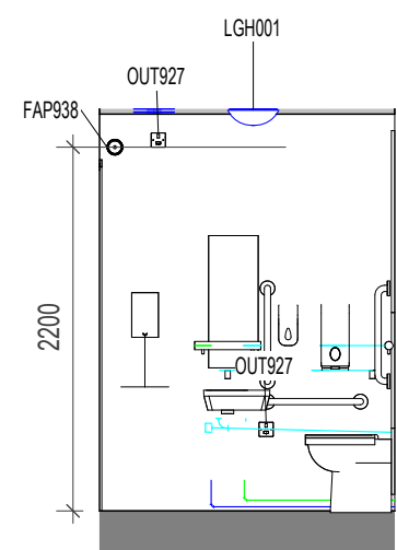
13 ELEVATION 13 1 : 50
