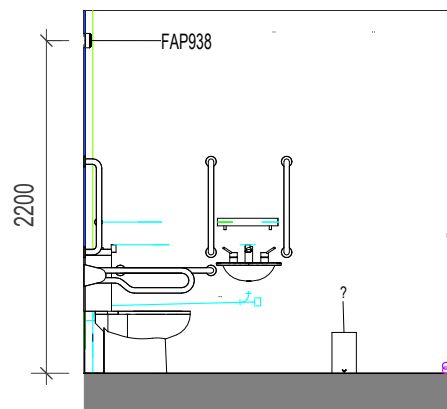
3 ELEVATION 3 1 : 50
