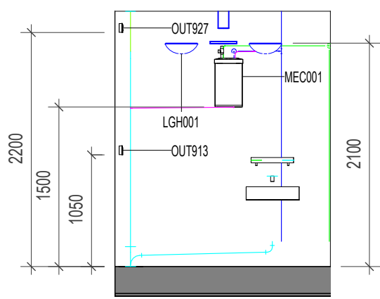
10 ELEVATION 10 1 : 50
