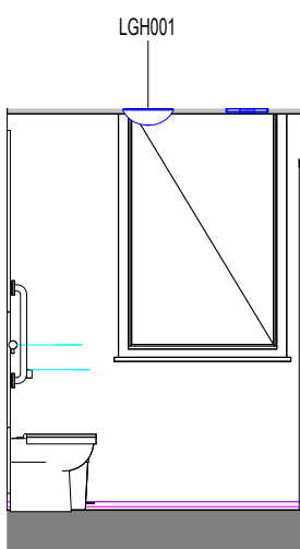
11 ELEVATION 11 1 : 50
