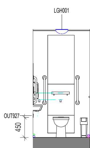
14 ELEVATION 14 1 : 50
