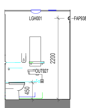
21 ELEVATION 21 1 : 50
