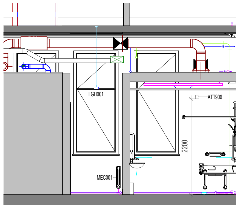
4 ELEVATION 4 1 : 50
