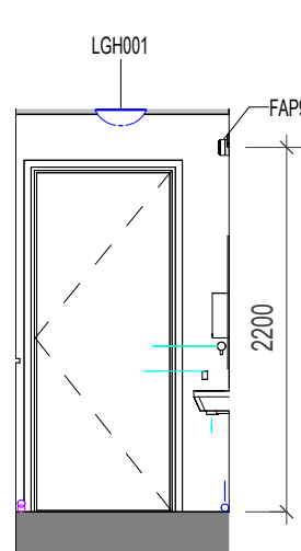
12 ELEVATION 12 1 : 50
