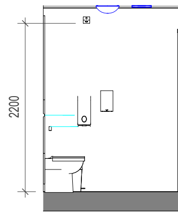
15 ELEVATION 15 1 : 50
