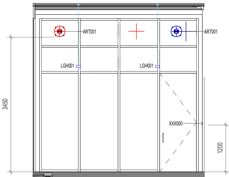
4 ELEVATION 4 1 : 50
