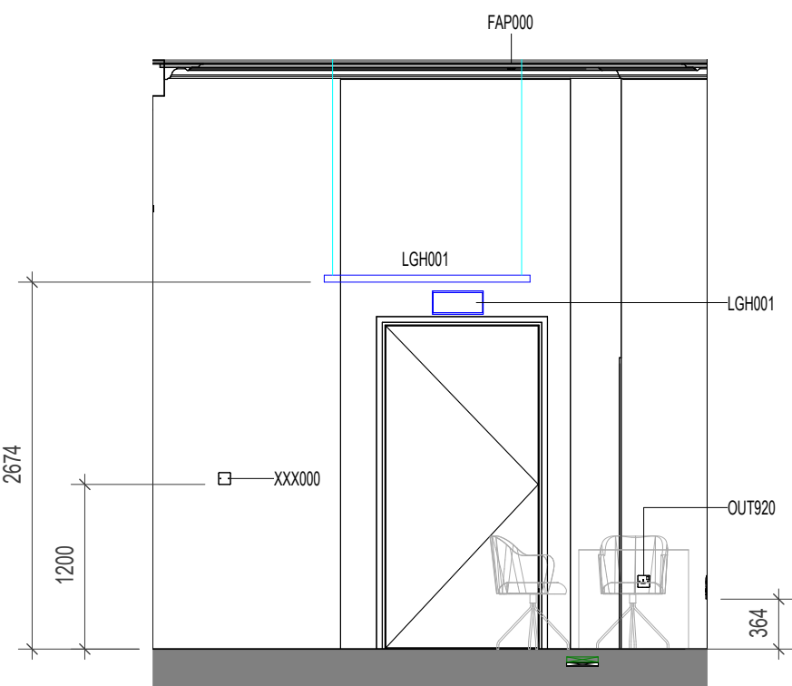
5 ELEVATION 5 1 : 50
