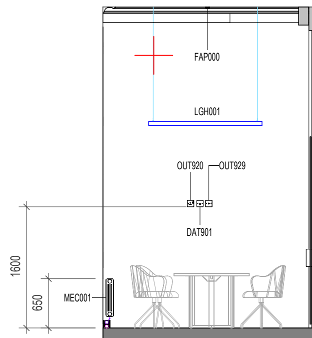
8 ELEVATION 8 1 : 50
