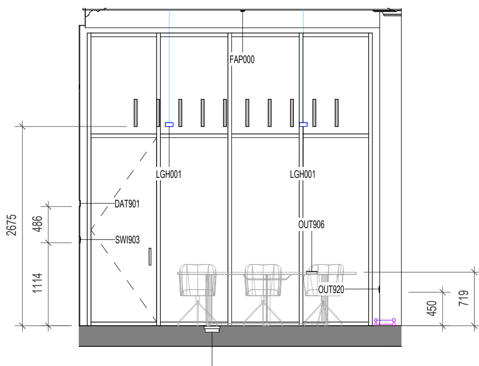
9 ELEVATION 9 1 : 50
