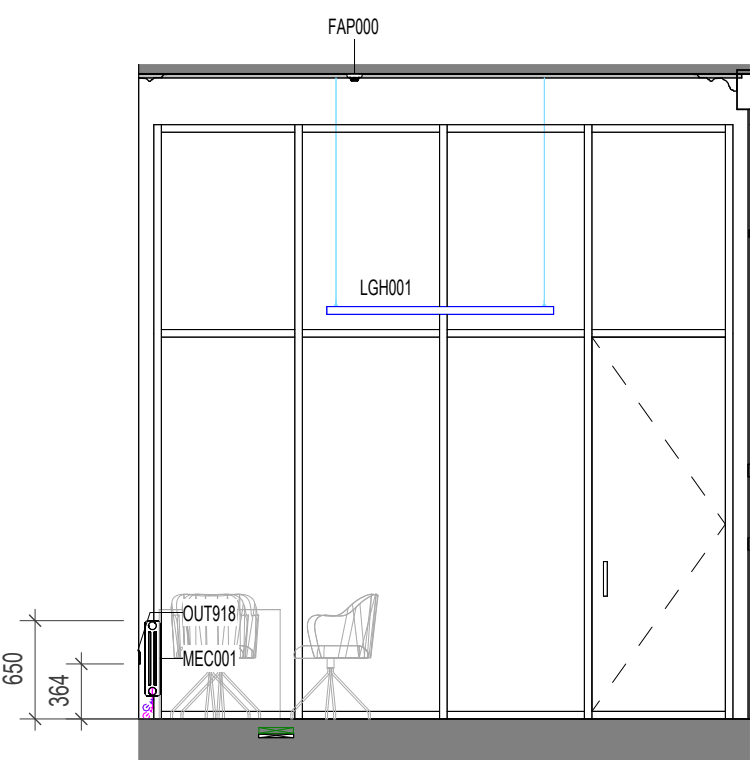
3 ELEVATION 3 1 : 50
