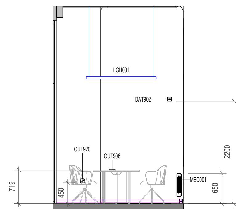
10 ELEVATION 10 1 : 50
