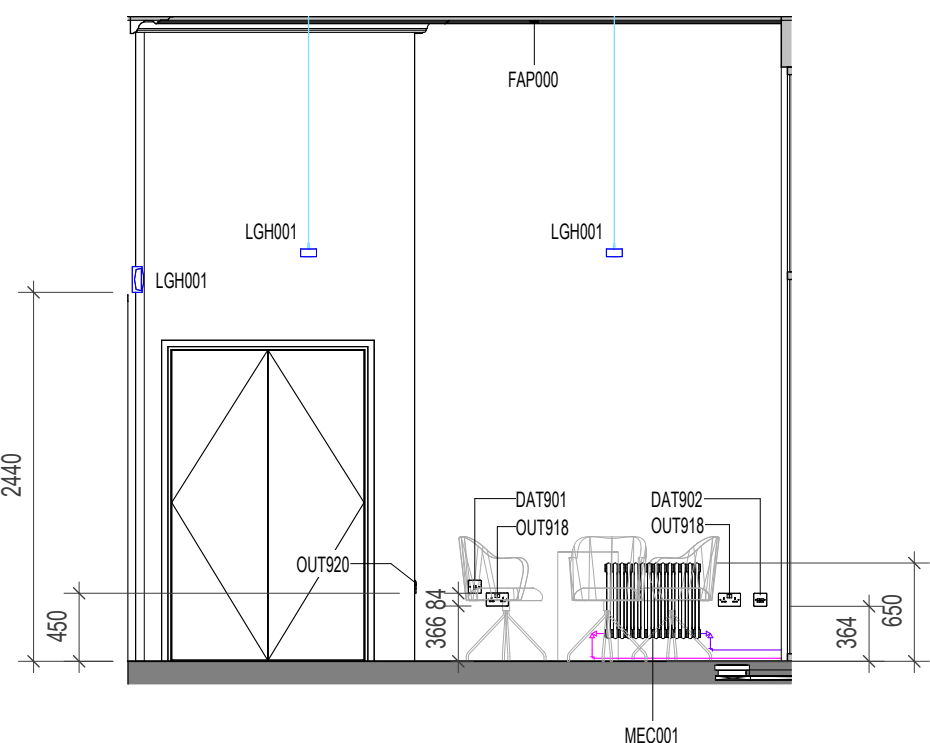
6 ELEVATION 6 1 : 50
