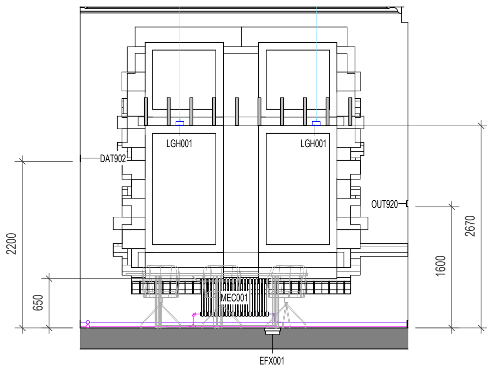
7 ELEVATION 7 1 : 50
