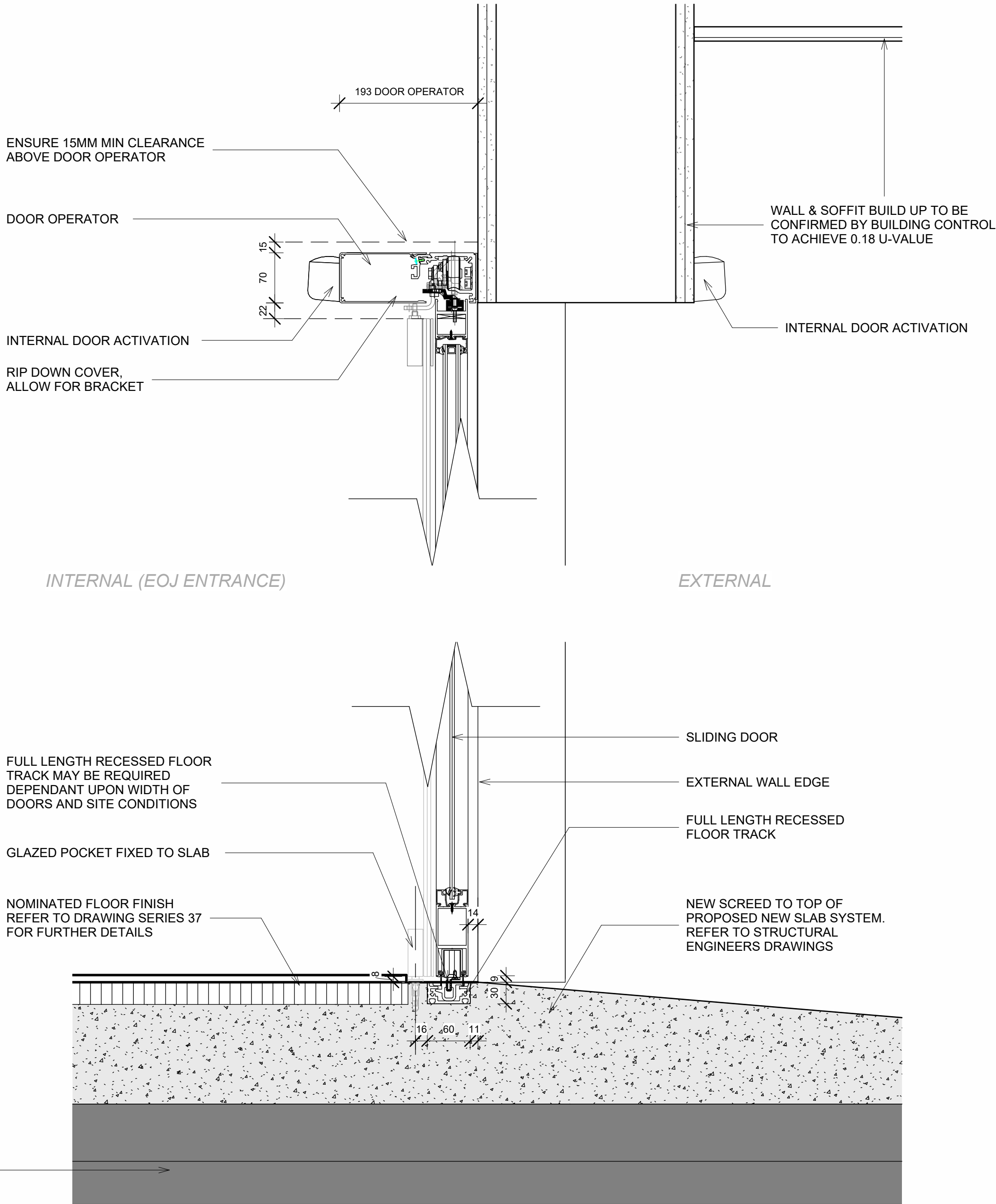
EOJ ENTRANCE DOOR SECTION A 1 : 5
