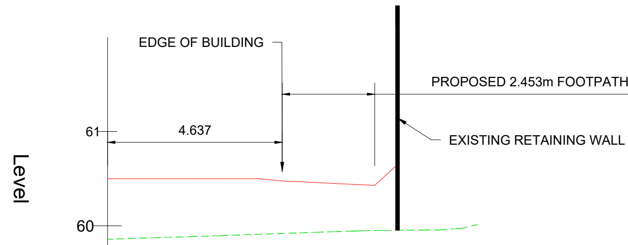
SECTION D-D - LONGSECTION SCALE: H 1:100,V 1:40. DATUM: 59.000
