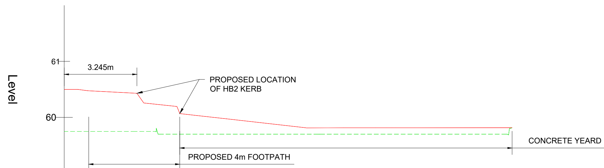
SECTION F-F - LONGSECTION SCALE: H 1:100,V 1:40. DATUM: 59.000
