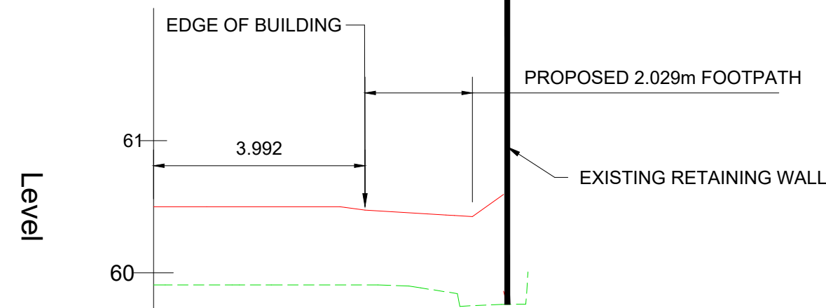
SECTION E-E - LONGSECTION SCALE: H 1:100,V 1:40. DATUM: 59.000
