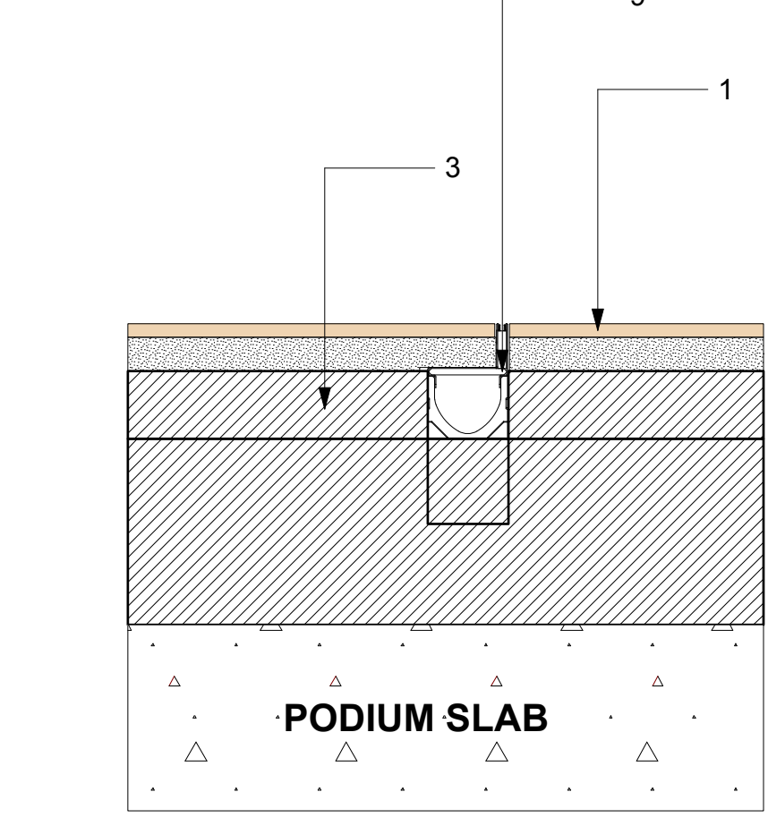
4 Slot Drain Scale: 1:10
