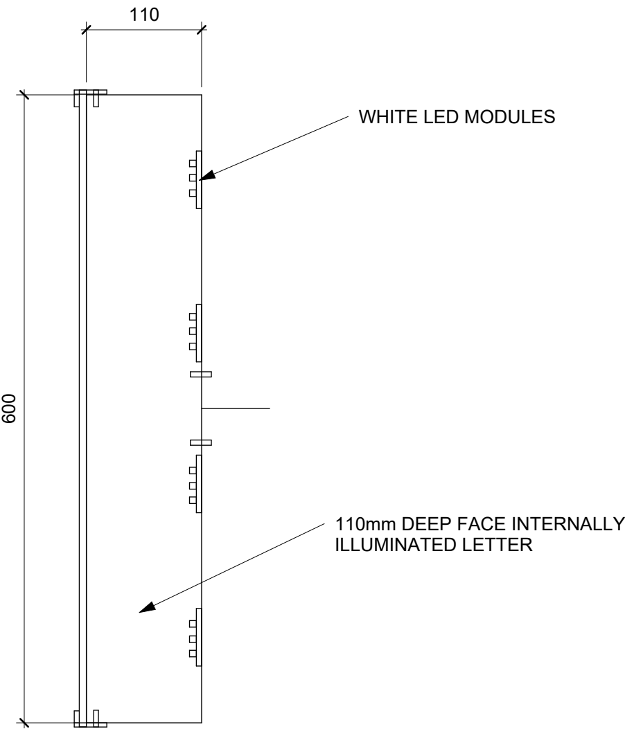
01 BLUE SAKURA LETTERS 1 : 5
