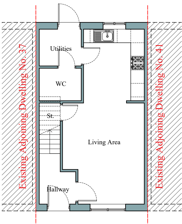
Existing G/F Plan 1:100
