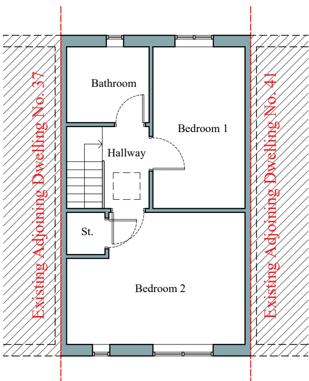
Existing 1/F Plan 1:100
