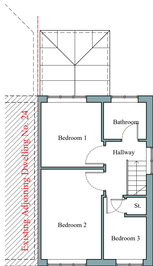
Existing 1/F Plan 1:100
