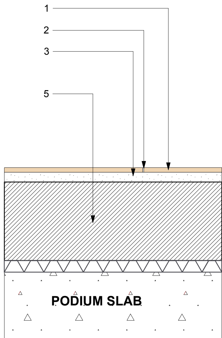
2 Build Up Void Forma Scale: 1:10
