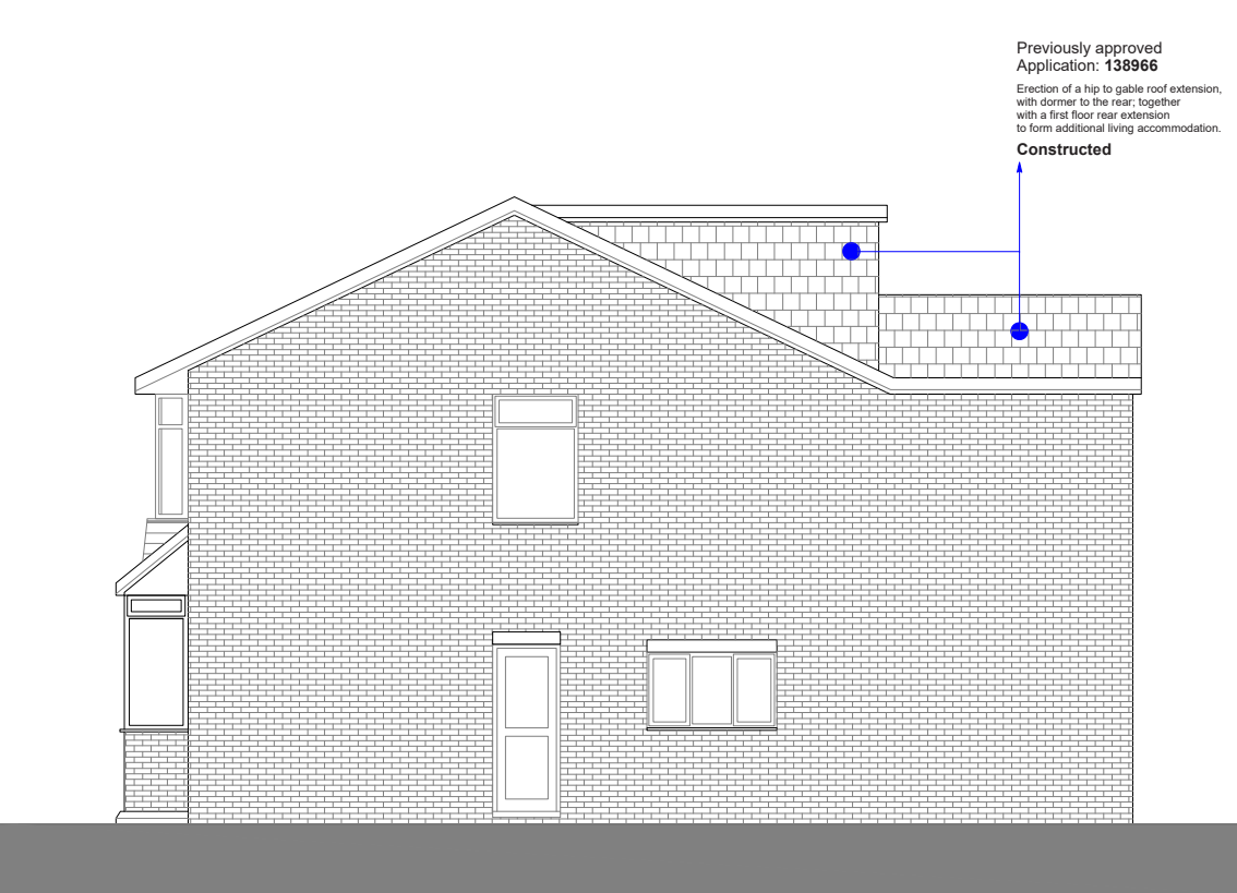
Existing Side Elevation 1:100 A3
