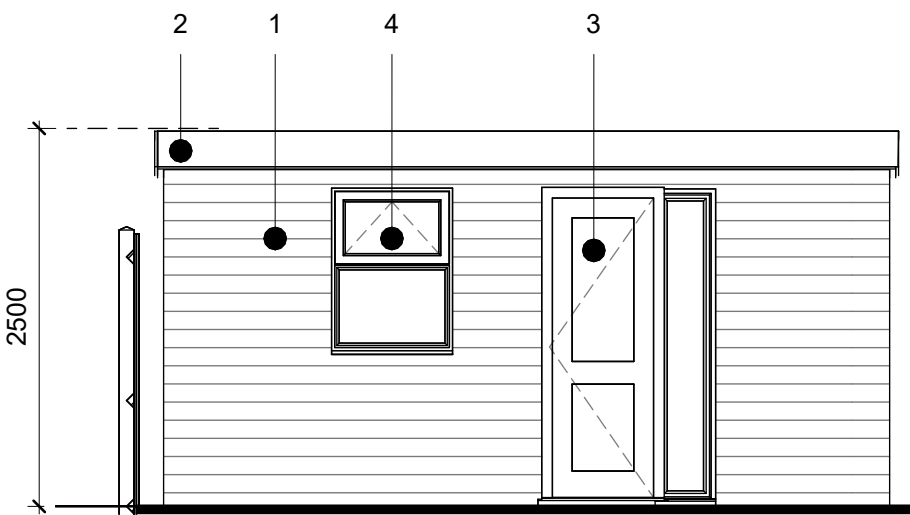
2 Elevation 1 - a 1 : 50
