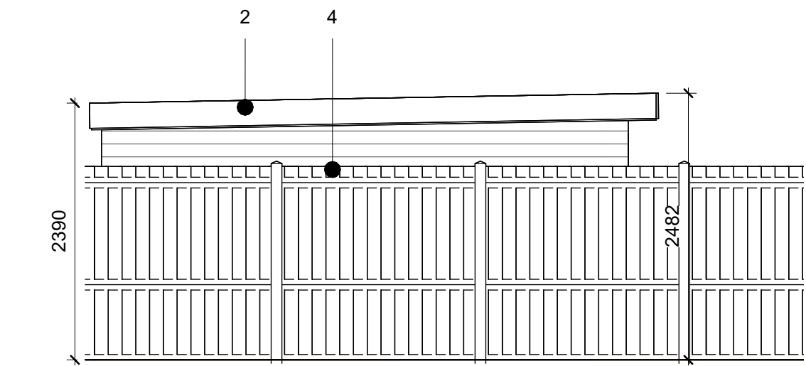
3 Elevation 2 - a 1 : 50
