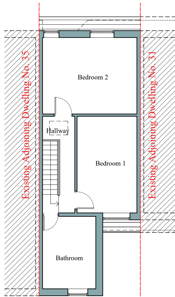
Existing 1/F Plan 1:100
