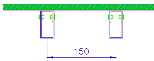
Typical Centres - GL Af & Ae - Fins
