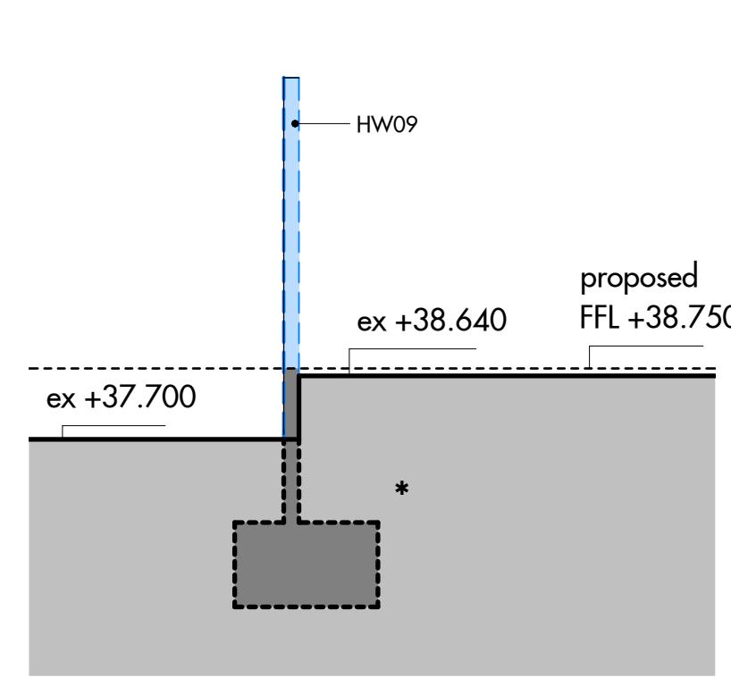
11 Holloway Wall Fabric Alterations Section DD 1 : 100
