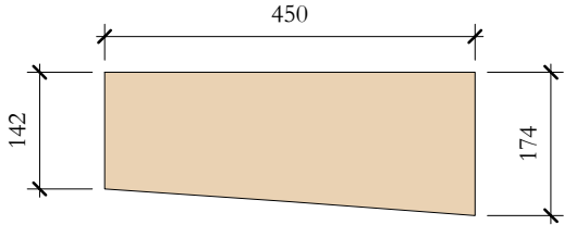
TcR_33 Elevation Top 1 : 10
