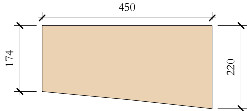
TcR_34 Elevation Top 1 : 10
