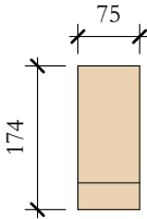
TcR_33 Elevation Left 1 : 10
