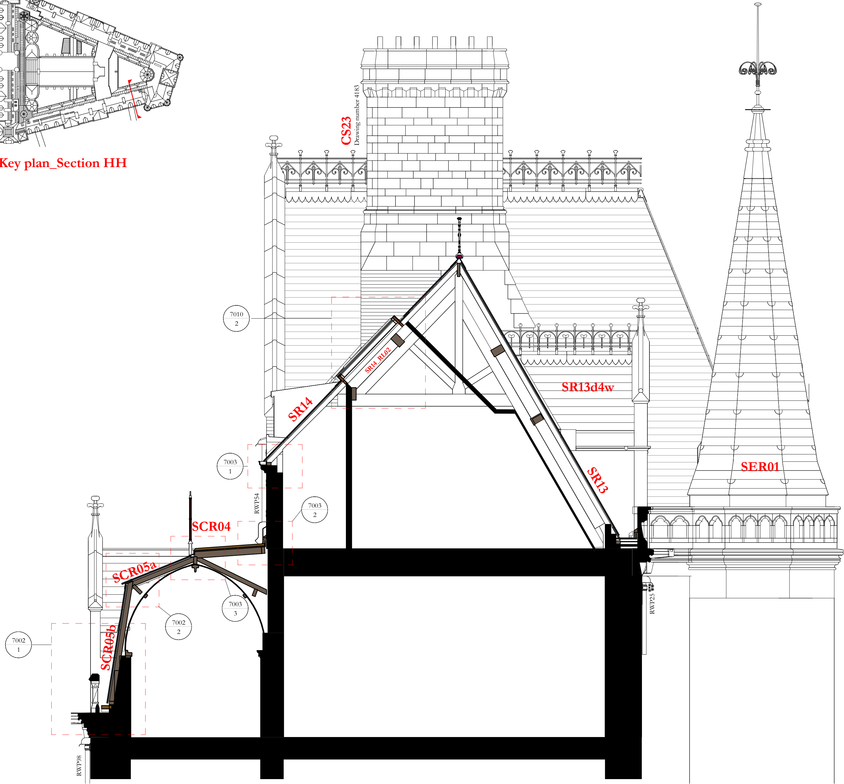
Section HH 1 : 50
