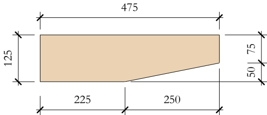
TcW_05 Elevation Top 1 : 10
