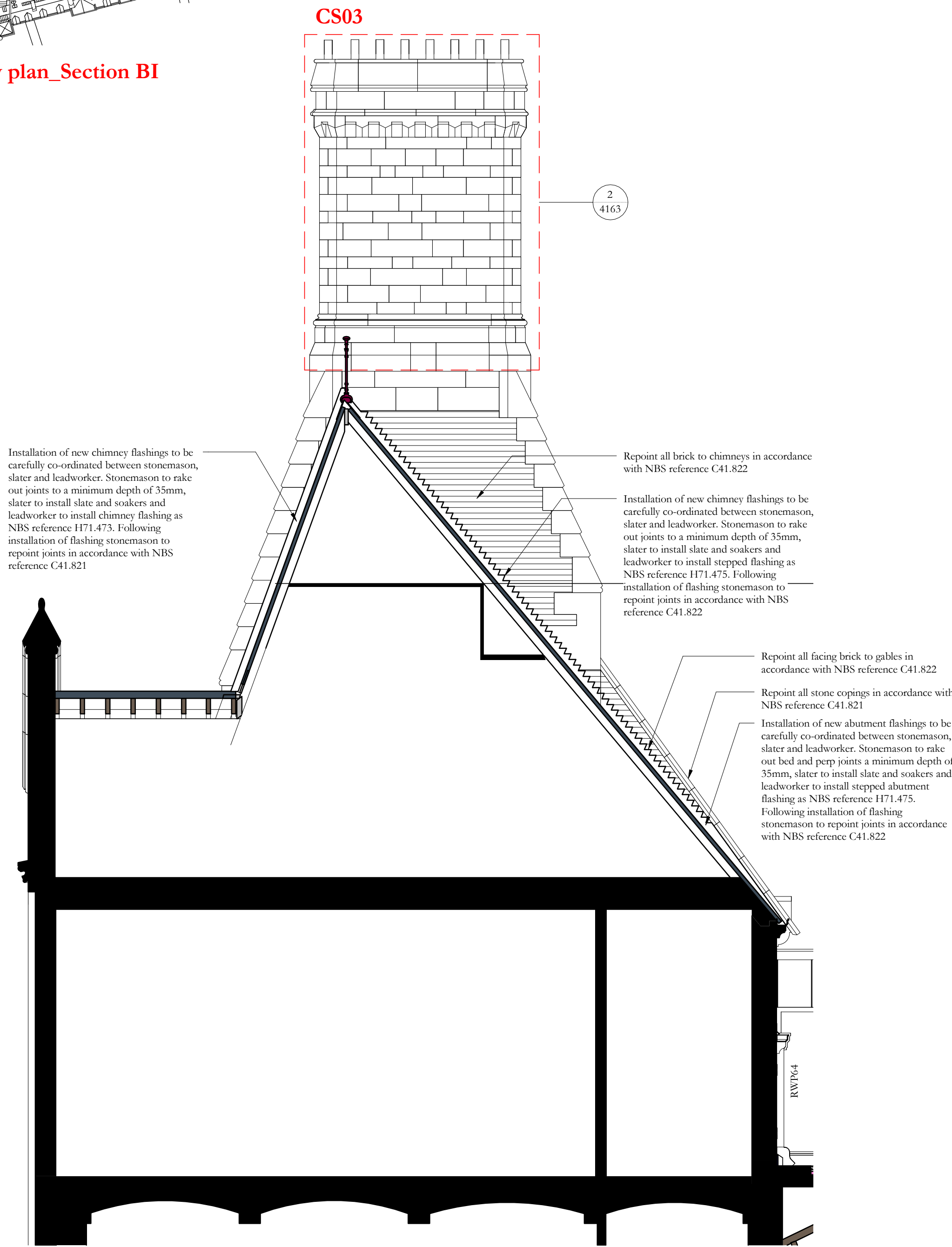
Section BI
