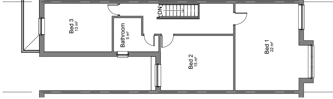
01-E-First Floor 1 : 100
