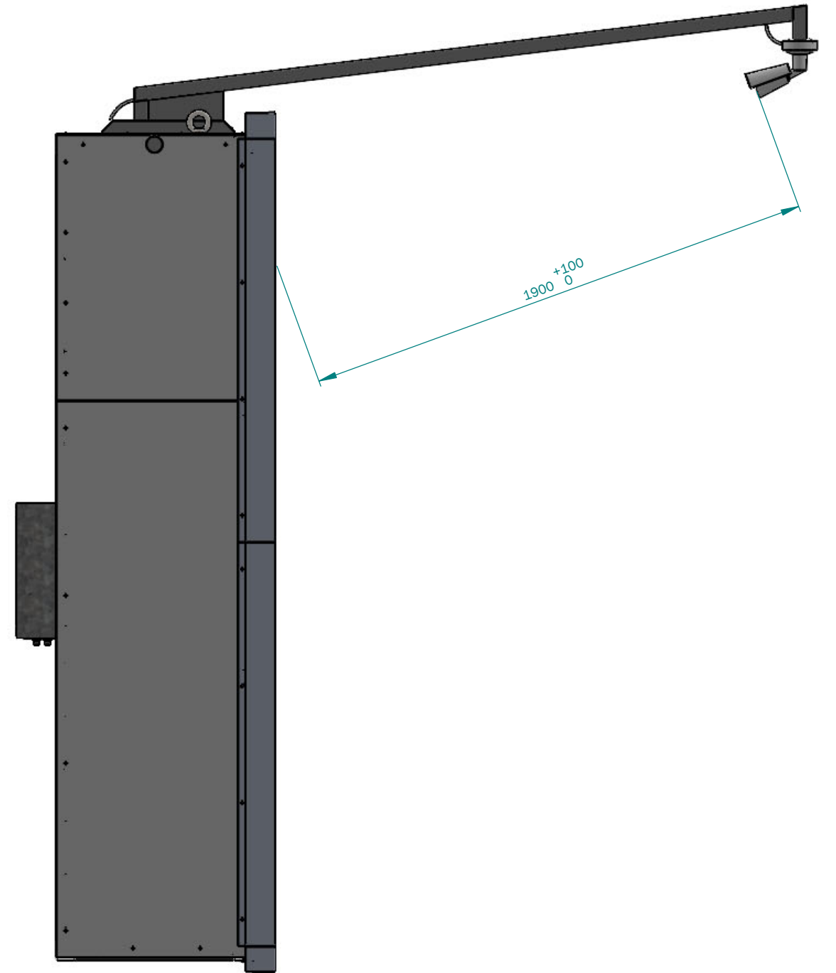
SIDE ELEVATION SCALE_1 : 20
