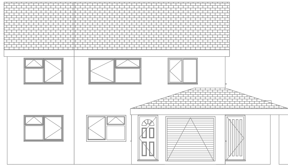
Front 1 : 100
