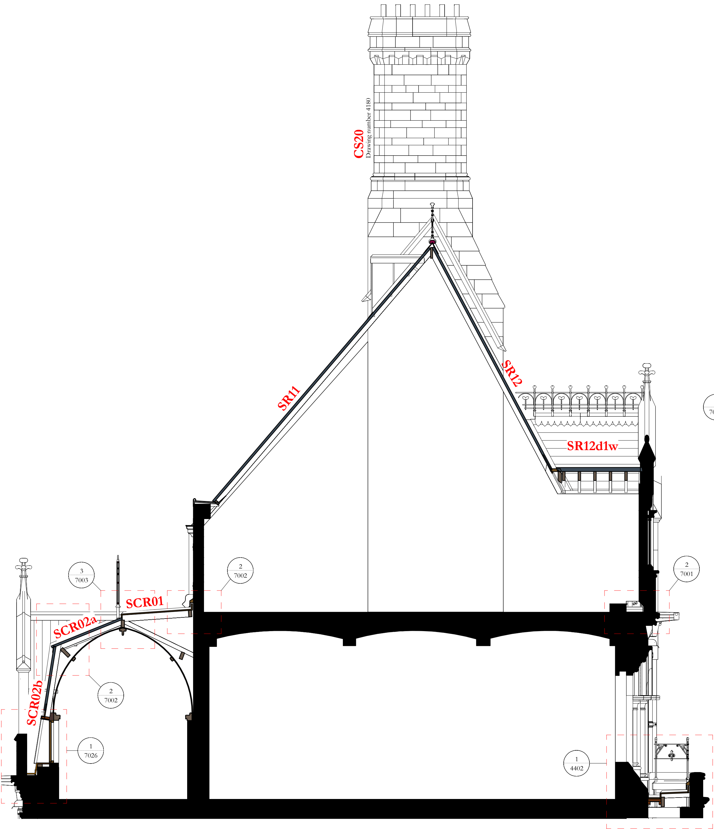
Section AC 1 : 50
