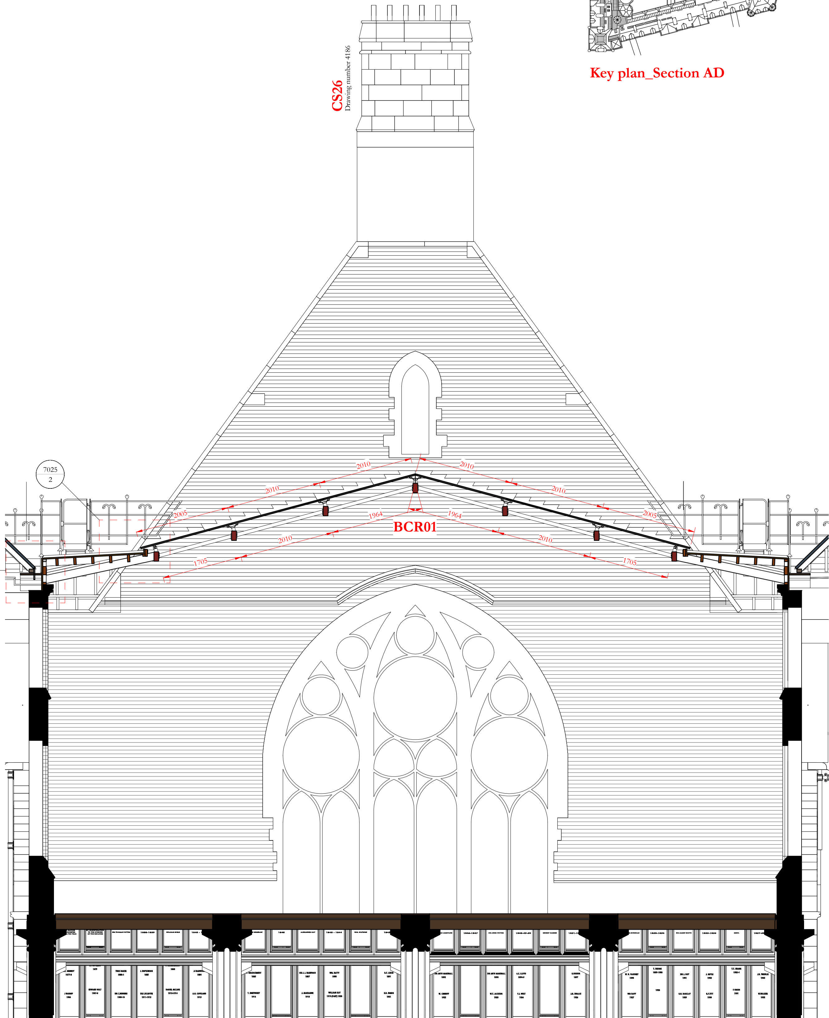
Section AD 1 : 50
