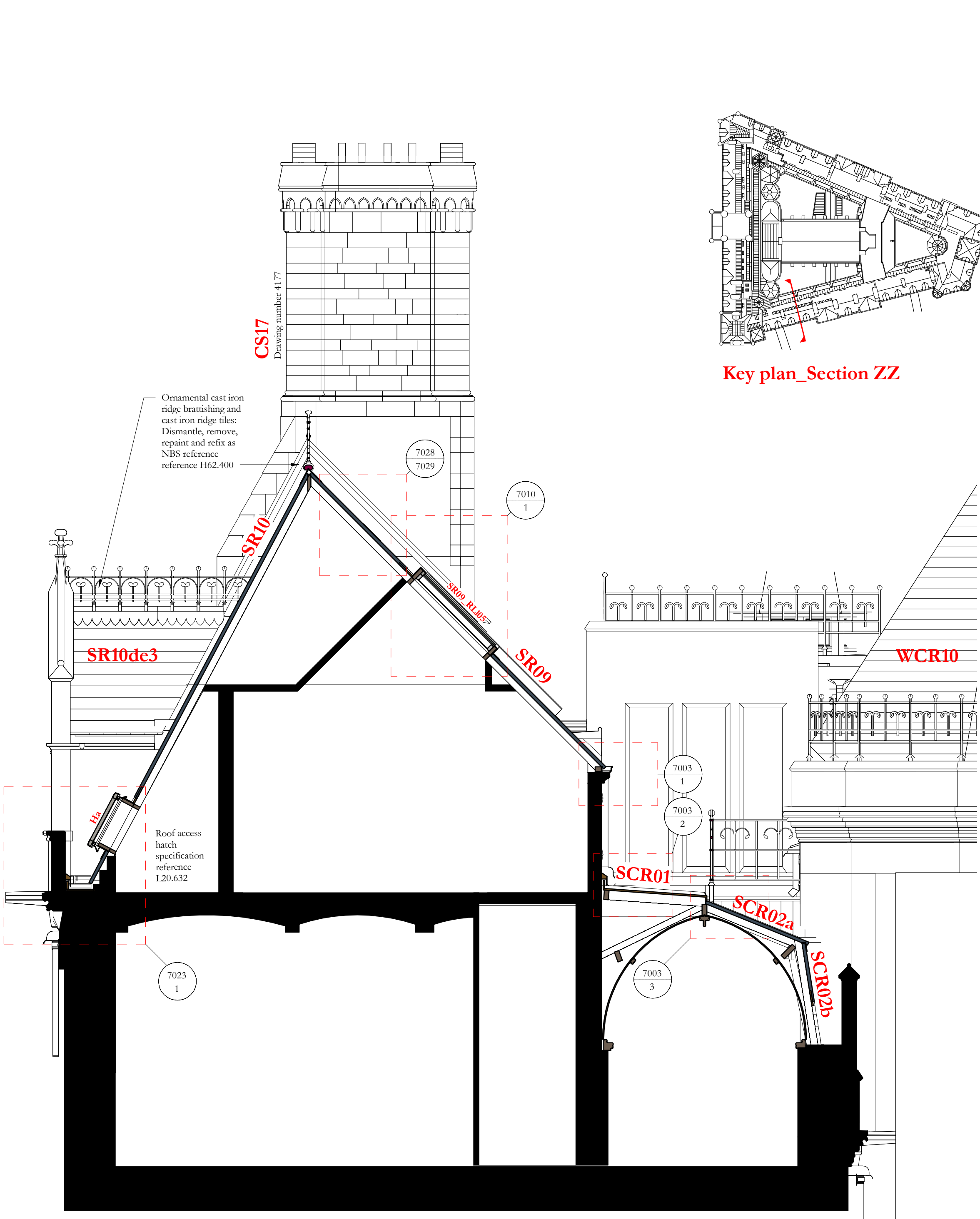
Section ZZ 1 : 50
