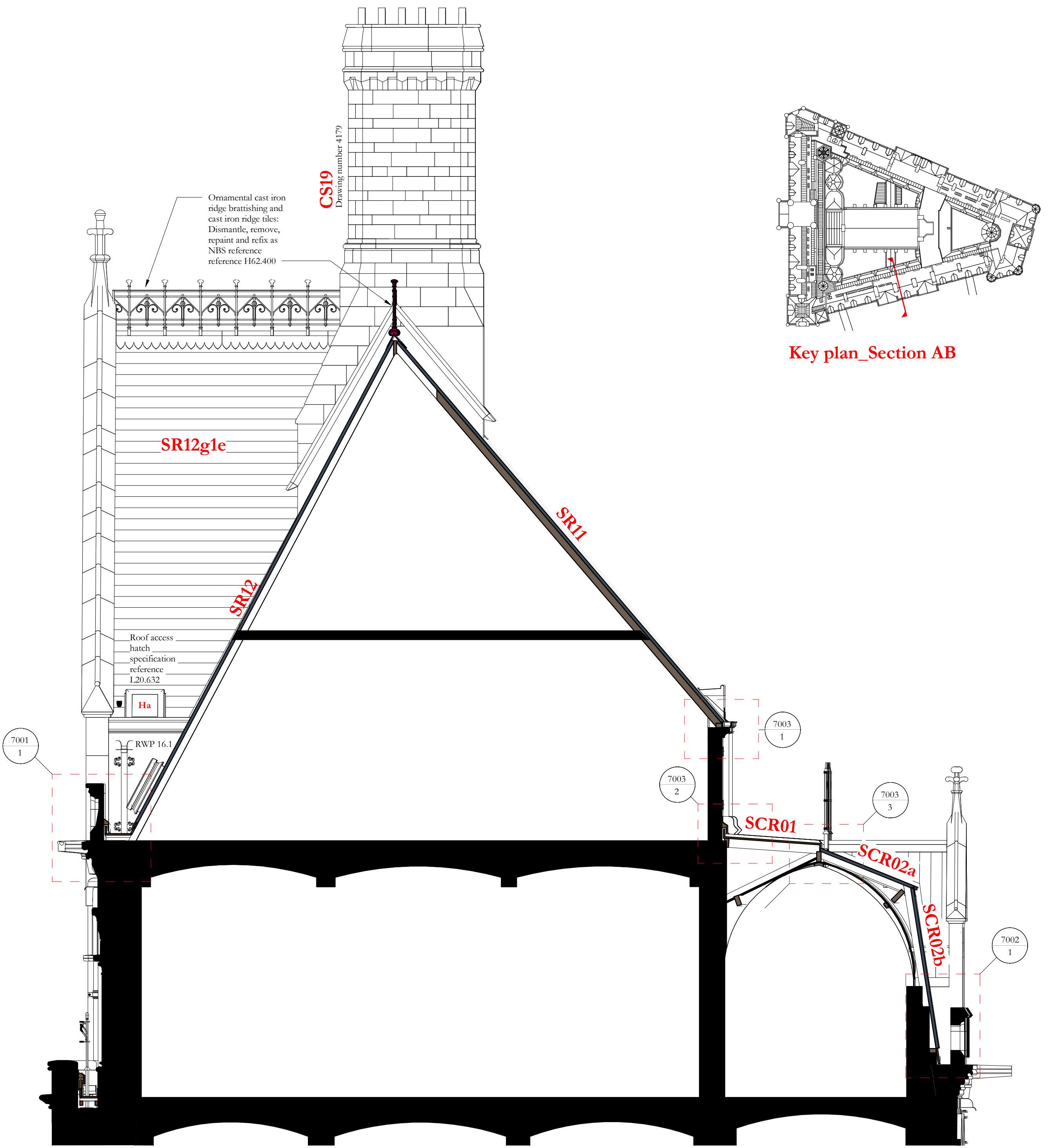
Section AB 1 : 50
