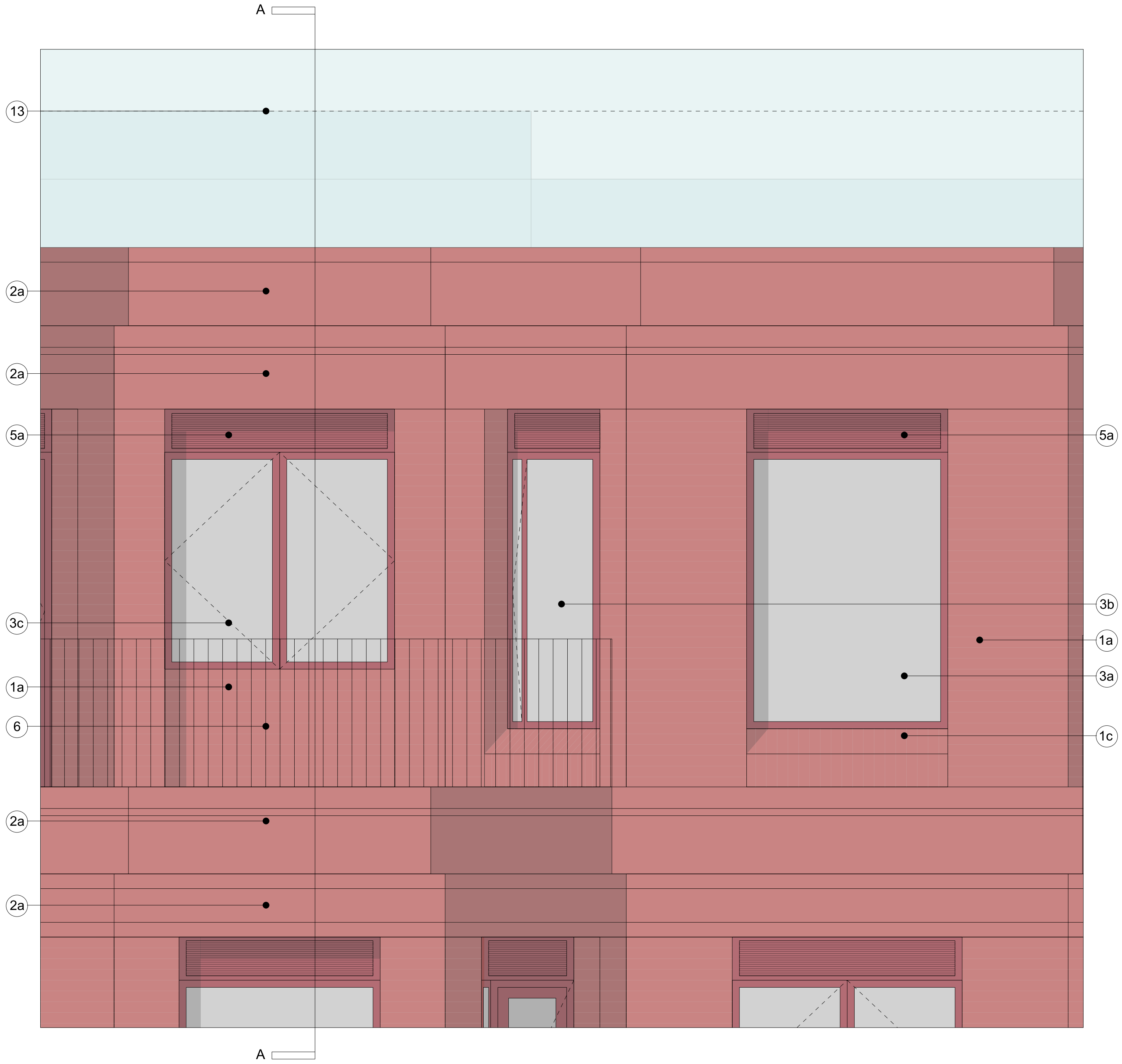
02 Elevation 1:20 @ A1
