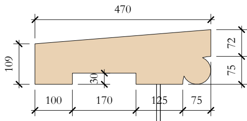
TcC_14 Elevation Left 1 : 10
