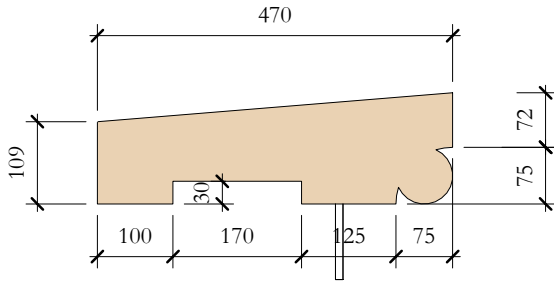
TcC_13 Elevation Left 1 : 10
