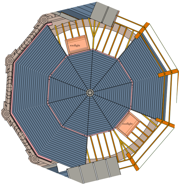
10a Plan Area 10 1 : 50
