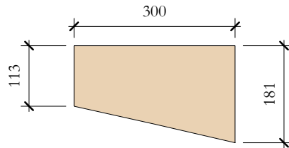
TcR_24 Elevation Top 1 : 10
