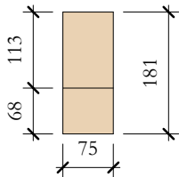
TcR_24 Elevation Left 1 : 10
