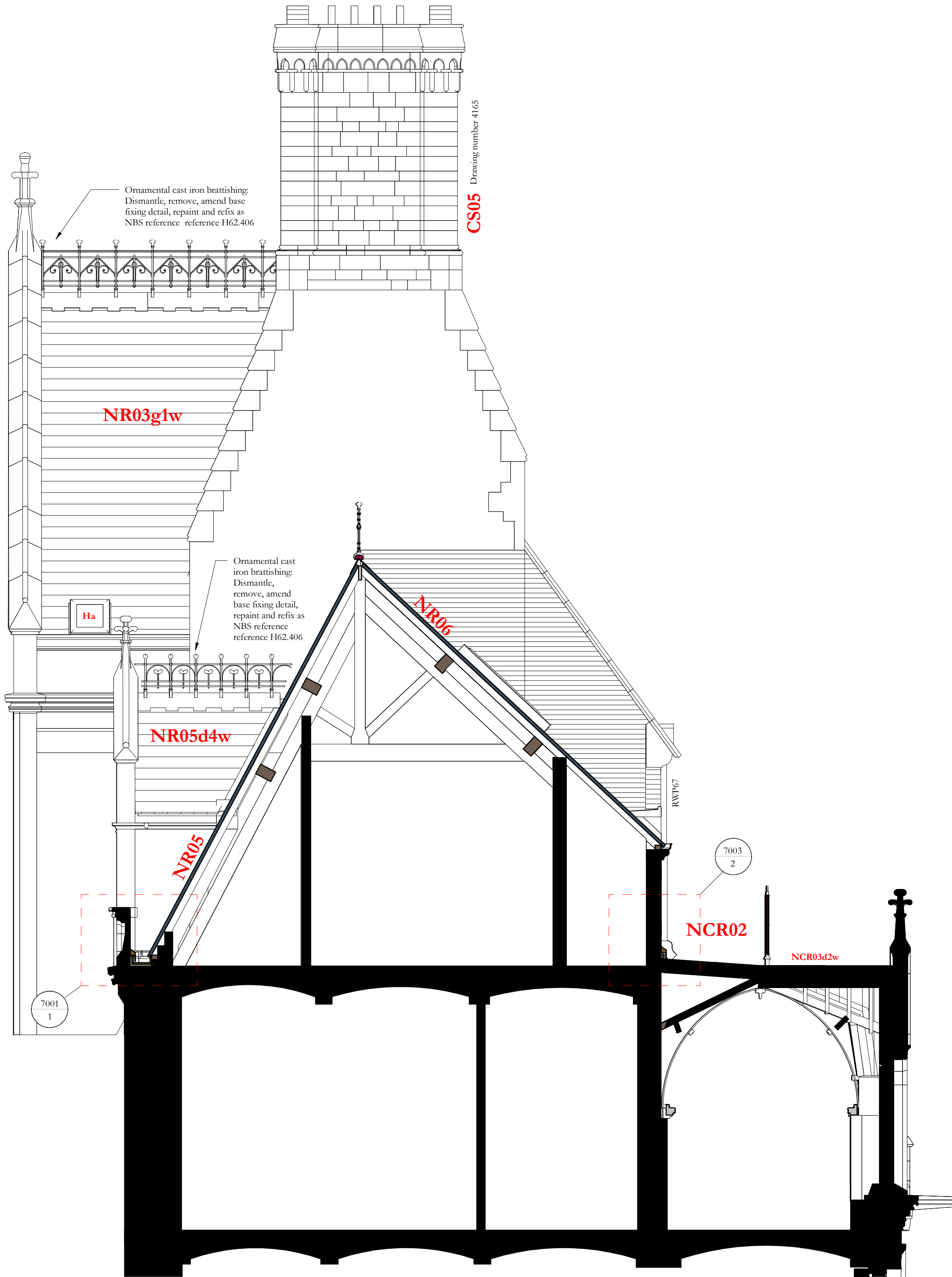
Section MM 1 : 50
